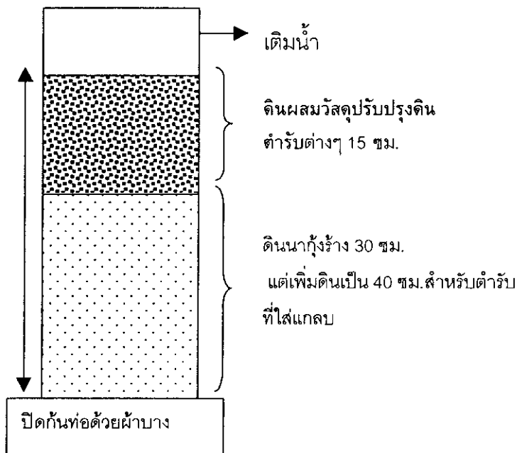
ภาพประกอบที่ 1 การเตรียมตัวอย่างทดลองในห้อง PVC เพื่อทดลองการระเหยน้ำและการกระจายเกลือในดินนาุ้งร้าง
