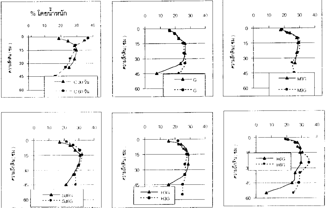
ภาพประกอบที่ 1 การกระจายความชื้นในดินตามความลึกของดินดำรับต่างๆ เมื่อสิ้นสุดการทดลอง 30 วัน (เส้นทึบ) และ 60 วัน (เส้นประ) โดย 15 ซม.ของดินบนเป็นดินผสม ส่วนดินล่างเป็นดินนาุ้งร้าง
