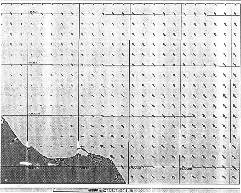
รูป E4.4 ขนาดและทิศทางของกระแสน้ำในเดือนกรกฎาคม ตลอดแนวท่อ (ต่อ)
