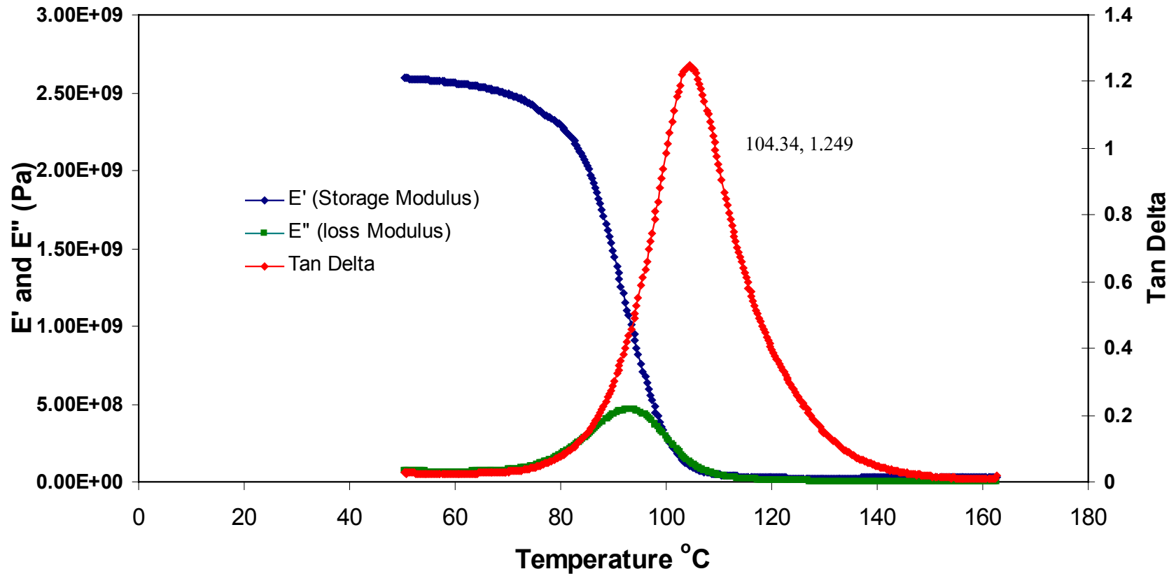
ภาพประกอบ 1 กราฟจากเครื่อง DMTA ความถี่ 1 Hz ของอีพ็อกซีสูตร I อบในเตาอบอุณหภูมิ 150 °C เวลา 14 นาที
