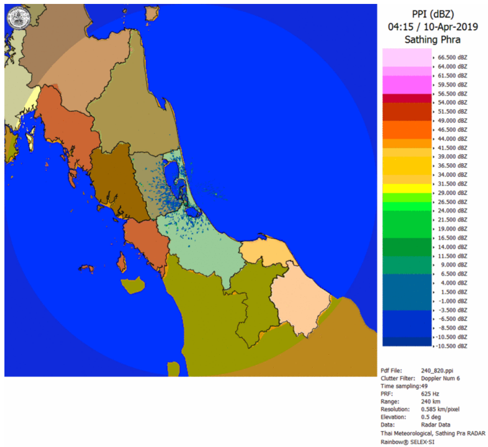
ภาพเรดาร์ตรวจอากาศ “สathingพระ” ณ วันที่ 10 เมษายน 2562 (ที่มา : กรมอุตุนิยมวิทยา)
