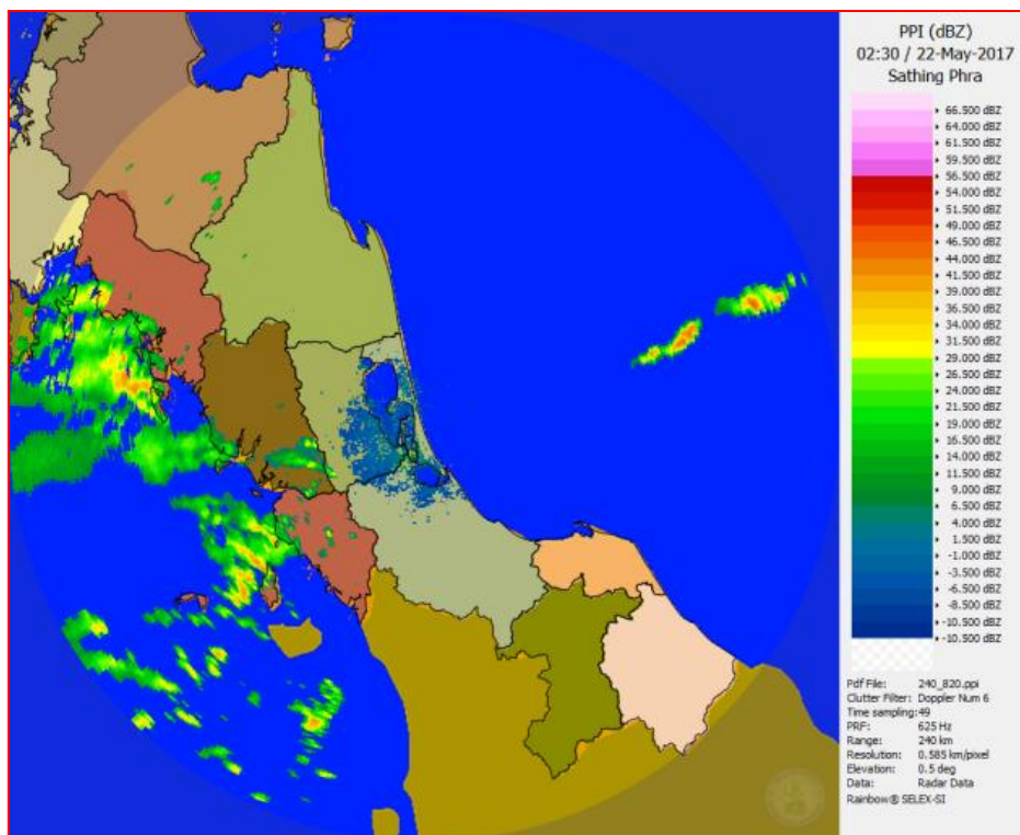
ภาพเรดาร์ตรวจอากาศ “สทิงพระ” ณ วันที่ 22 พฤษภาคม 2560 (ที่มา : กรมอุตุนิยมวิทยา)
