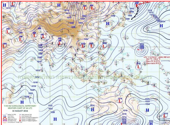
แผนที่อากาศ วันที่ 10 ส.ค. 2559 เวลา 07.00 น.
