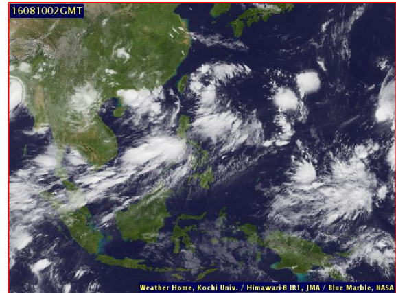
ภาพถ่ายจากดาวเทียม วันที่ 10 ส.ค. 2559
