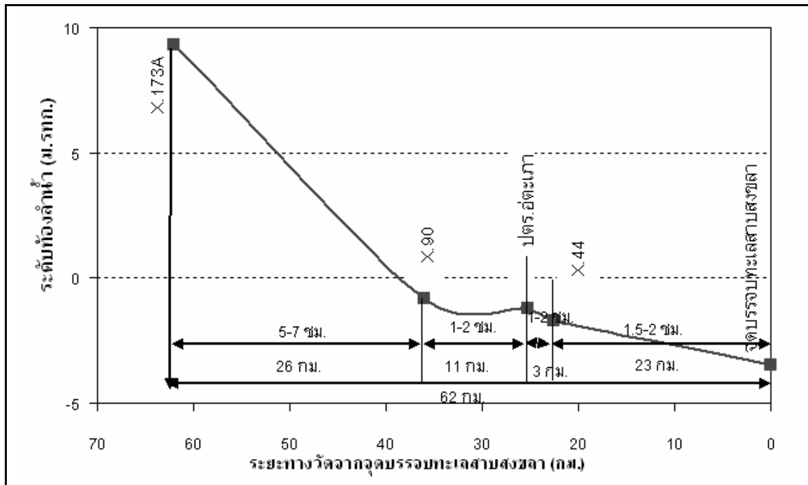
รูปที่ 4 รูปตัดตามยาวและเวลาการเดินทางของน้ำในคลองอยู่ตะเภาดั้งแต่ สถานีหน้าท่า X.173A ถึงจุดบรรจบทะเลสาบสงขลา
