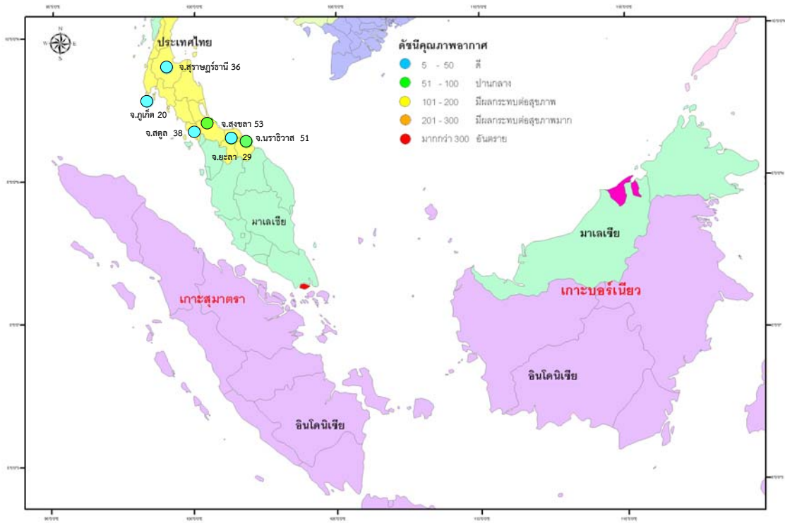
รูปที่ 3 ดัชนีคุณภาพอากาศ วันที่ 19 สิงหาคม 2556 (เนื่องจากสถานีขัดข้อง ข้อมูลคุณภาพอากาศของ จังหวัดนราธิวาส และสงขลา เป็นข้อมูลเมื่อวันที่ 16 และ 17 สิงหาคม 2556ตามลำดับ)
