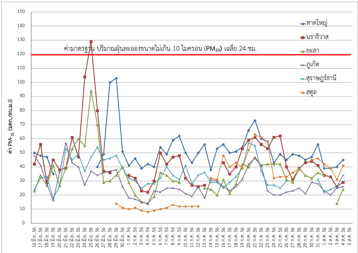
รูปที่ 5 แสดงการเปลี่ยนแปลงของปริมาณฝุ่นละอองขนาดไม่เกิน 10 ไมครอน (PM10) ระหว่างวันที่ 16 มิถุนายน - 4 สิงหาคม 2556
