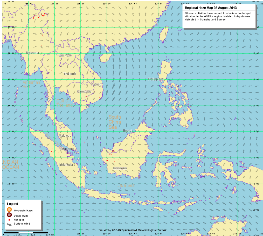
รูปที่ 2 ทิศทางลม เมื่อวันที่ 3 สิงหาคม 2556
