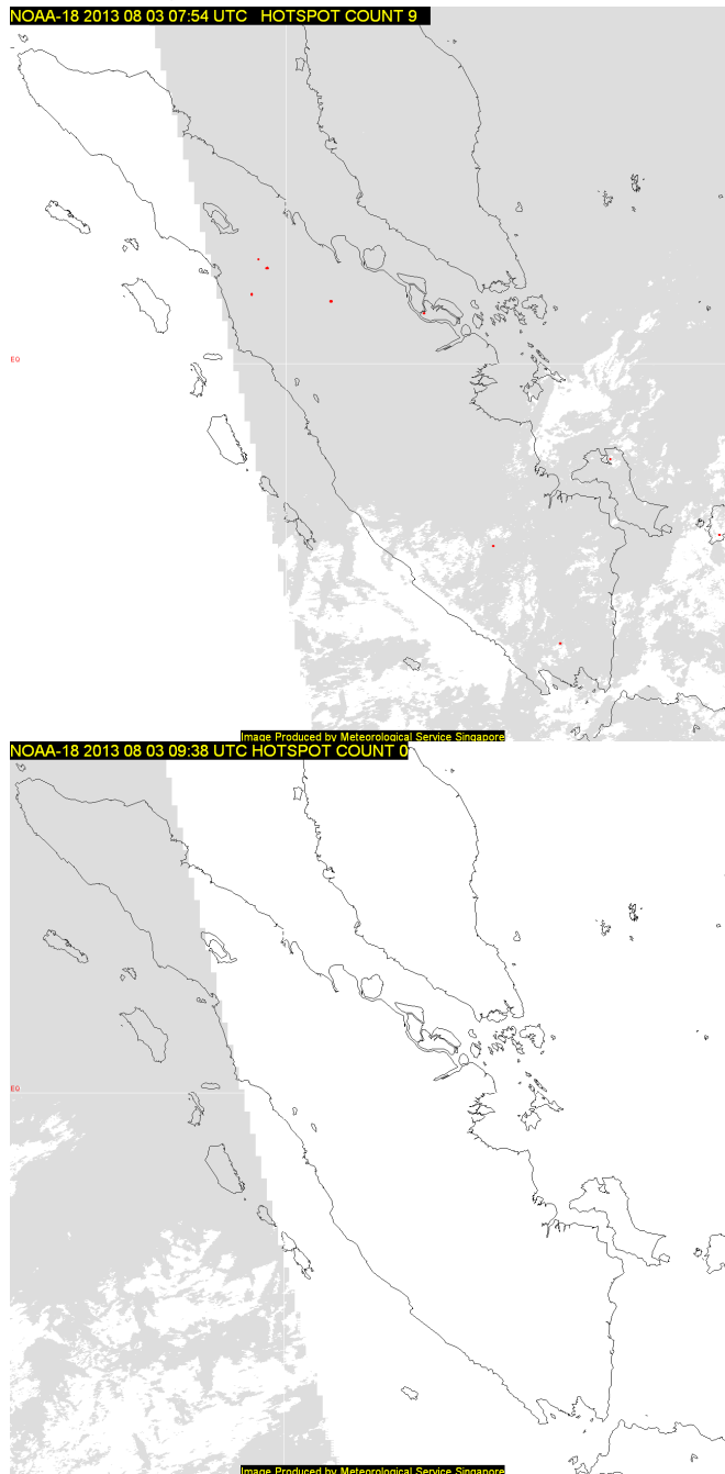
รูปที่ 1 จำนวนจุดที่เกิดไฟไหม้บนเกาะสุมาตรา เมื่อวันที่ 3 สิงหาคม 2556
