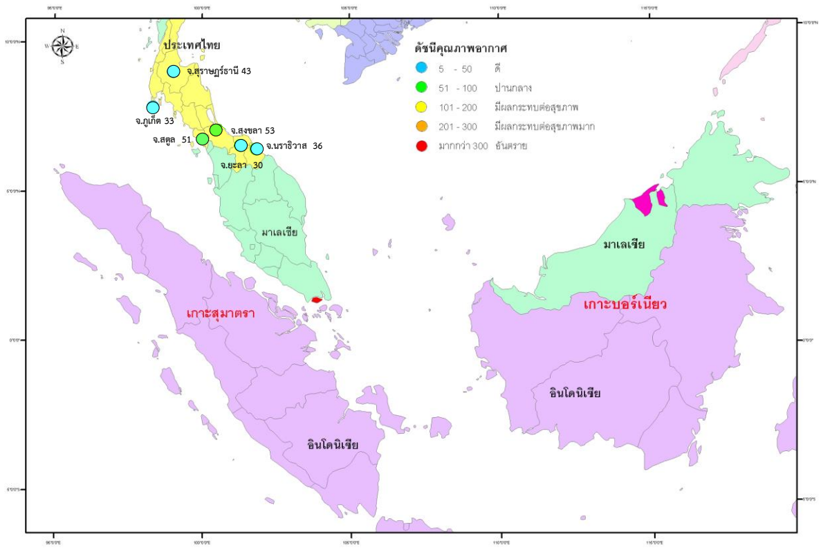
รูปที่ 3 ดัชนีคุณภาพอากาศ วันที่ 4 สิงหาคม 2556
