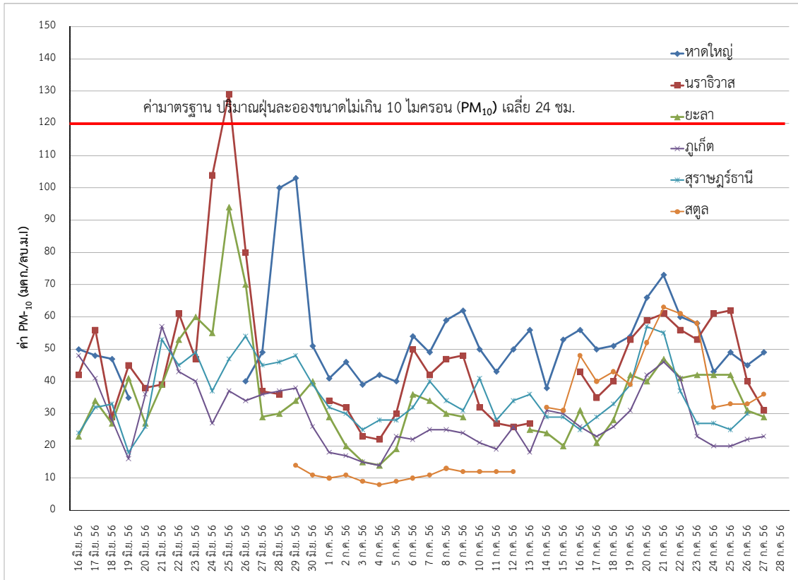
รูปที่ 5 แสดงการเปลี่ยนแปลงของปริมาณฝุ่นละอองขนาดไม่เกิน 10 ไมครอน (PM10) ระหว่างวันที่ 16 มิถุนายน - 27 กรกฎาคม 2556
