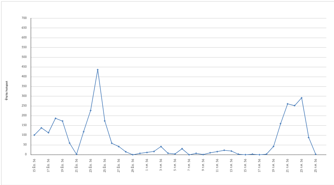
รูปที่ 4 แสดงการเปลี่ยนแปลงของ Hotspot บนเกาะสุมาตรา ระหว่างวันที่ 15 มิถุนายน - 25 กรกฎาคม 2556
