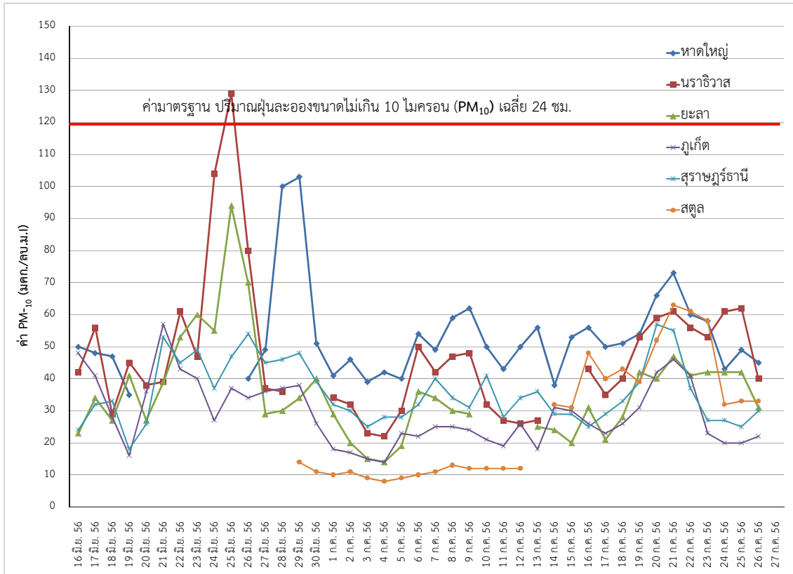
รูปที่ 5 แสดงการเปลี่ยนแปลงของปริมาณฝุ่นละอองขนาดไม่เกิน 10 ไมครอน (PM10) ระหว่างวันที่ 16 มิถุนายน - 26 กรกฎาคม 2556
