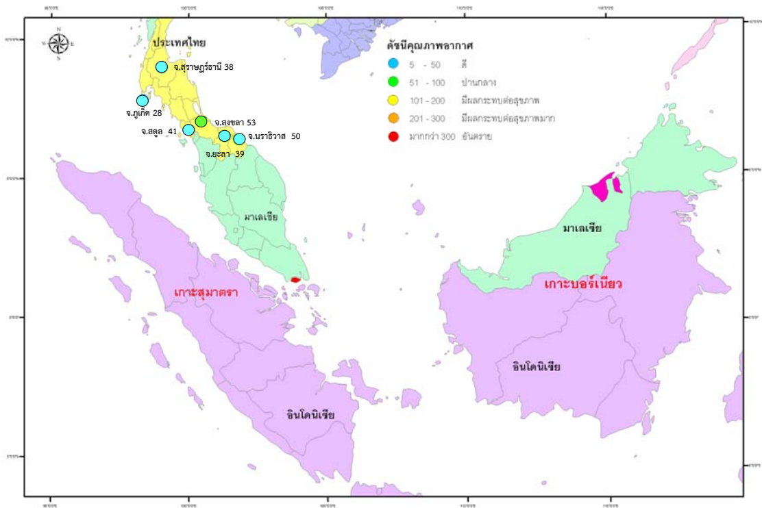
รูปที่ 3 ดัชนีคุณภาพอากาศ วันที่ 26 กรกฎาคม 2556
