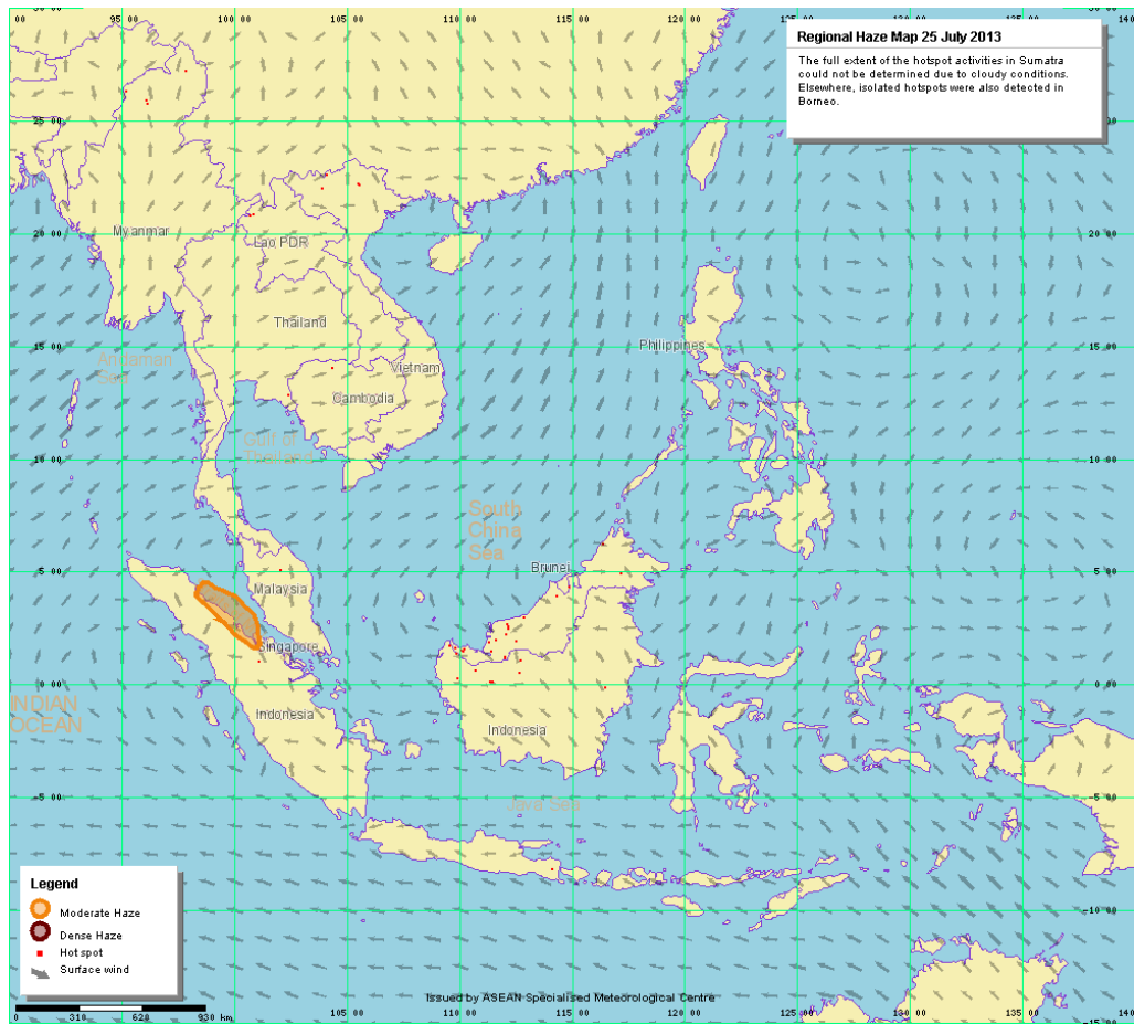
รูปที่ 2 ทิศทางลม เมื่อวันที่ 25 กรกฎาคม 2556
