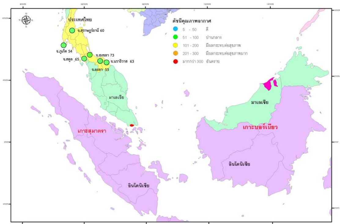
รูปที่ 3 ดัชนีคุณภาพอากาศ วันที่ 21 กรกฎาคม 2556
