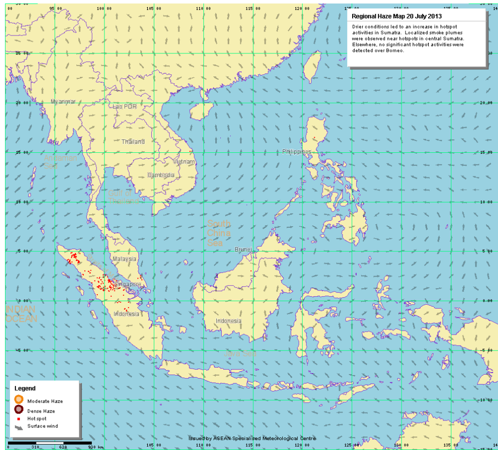
รูปที่ 2 ทิศทางลม เมื่อวันที่ 20 กรกฎาคม 2556
