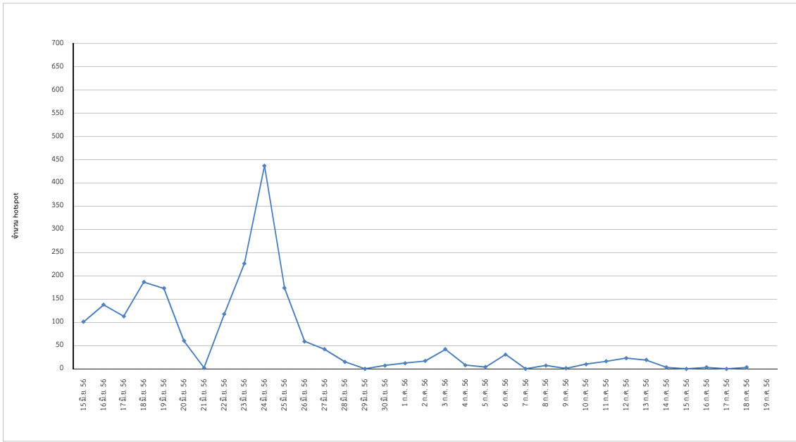
รูปที่ 4 แสดงการเปลี่ยนแปลงของ Hotspot บนเกาะสุมาตรา ระหว่างวันที่ 15 มิถุนายน - 18 กรกฎาคม 2556
