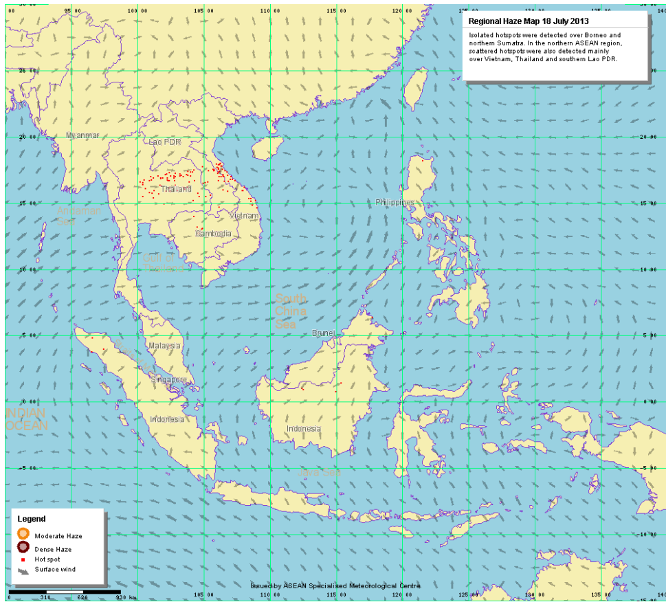
รูปที่ 2 ทิศทางลม เมื่อวันที่ 18 กรกฎาคม 2556
