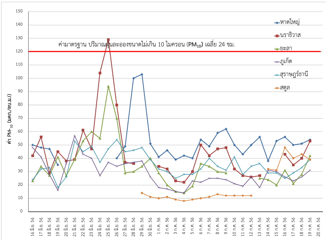
รูปที่ 5 แสดงการเปลี่ยนแปลงของปริมาณฝุ่นละอองขนาดไม่เกิน 10 ไมครอน (PM10) ระหว่างวันที่ 16 มิถุนายน - 19 กรกฎาคม 2556
