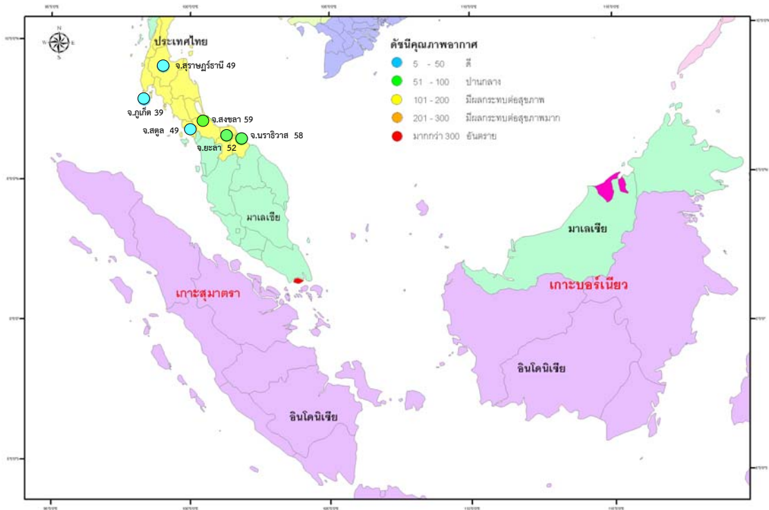
รูปที่ 3 ดัชนีคุณภาพอากาศ วันที่ 19 กรกฎาคม 2556
