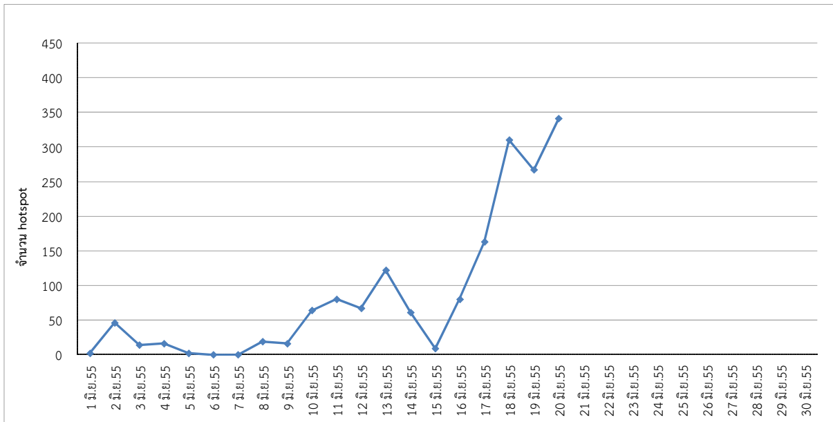
รูปที่ 4 แสดงการเปลี่ยนแปลงของจำนวน Hotspot บนเกาะสุมาตรา ระหว่างวันที่ 1-20 มิถุนายน 2555
