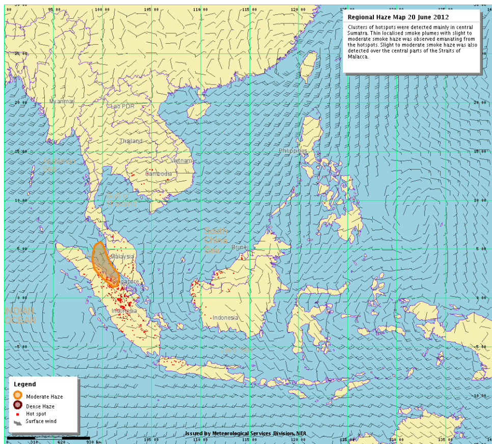
รูปที่ 2 ทิศทางลม เมื่อวันที่ 20 มิถุนายน 2555
