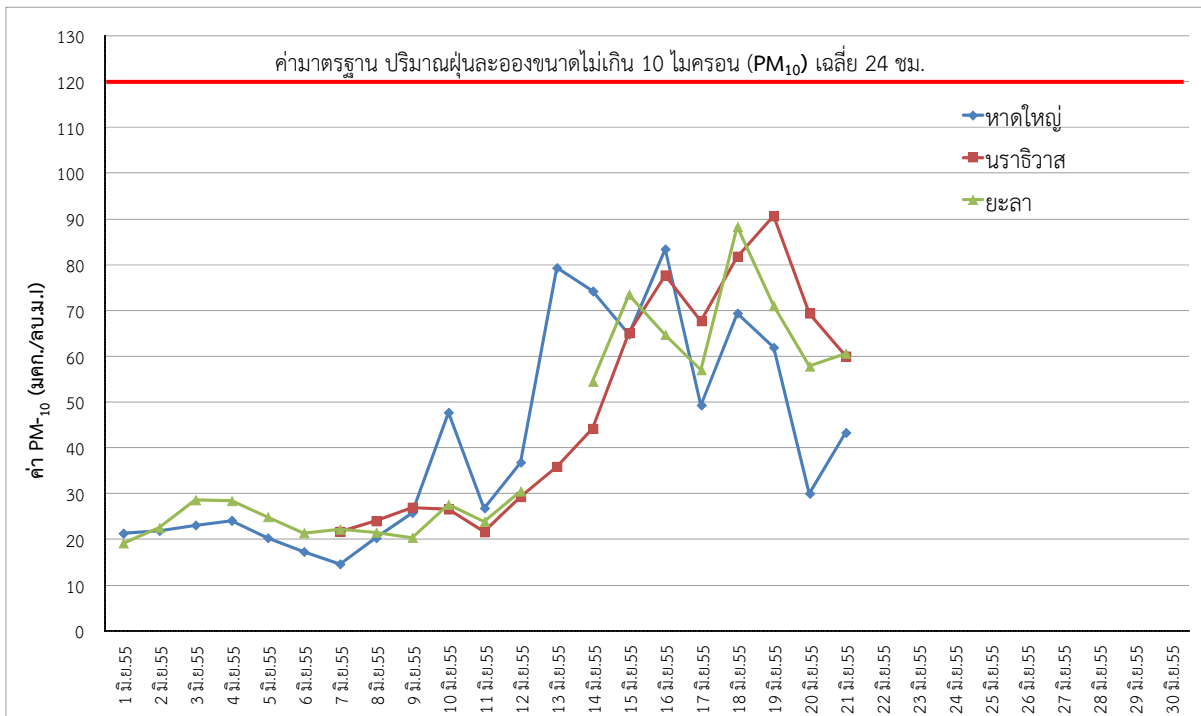
รูปที่ 5 แสดงการเปลี่ยนแปลงของปริมาณฝุ่นละอองขนาดไม่เกิน 10 ไมครอน (PM 10 ) ระหว่างวันที่ 1 - 21 มิถุนายน 2555
