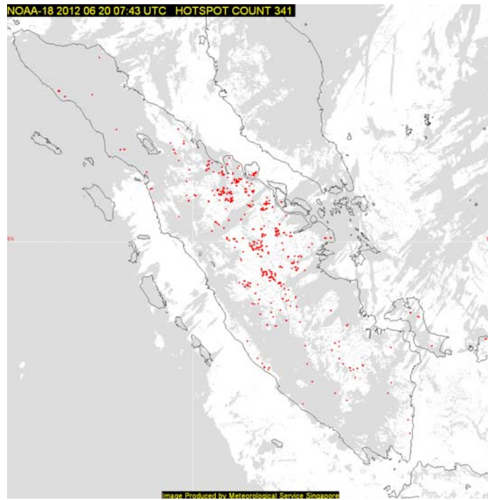
รูปที่ 1 จำนวนจุดที่เกิดไฟไหม้บนเกาะสุมาตรา ประเทศอินโดนีเซีย เมื่อวันที่ 20 มิถุนายน 2555
