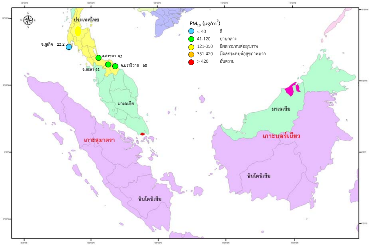
รูปที่ 3 แสดงค่าเฉลี่ยฝุ่นละอองขนาดไม่เกิน 10 ไมครอน ในเวลา 24 ชั่วโมง วันที่ 21 มิถุนายน 2555
