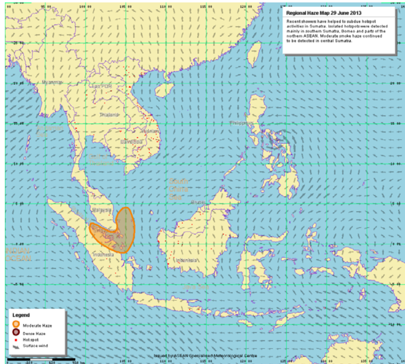
รูปที่ 2 ทิศทางลม เมื่อวันที่ 29 มิถุนายน 2556
