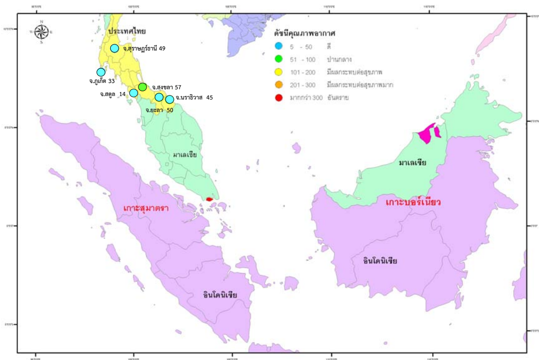
รูปที่ 3 ดัชนีคุณภาพอากาศ วันที่ 30 มิถุนายน 2556
