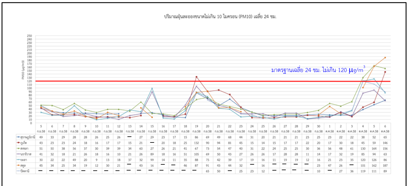
รูปที่ 5 แสดงการเปลี่ยนแปลงของปริมาณฝุ่นละอองขนาดไม่เกิน 10 ไมครอน (PM 10 ) ระหว่างวันที่ 5 ก.ย. – 6 ต.ค. 2558
