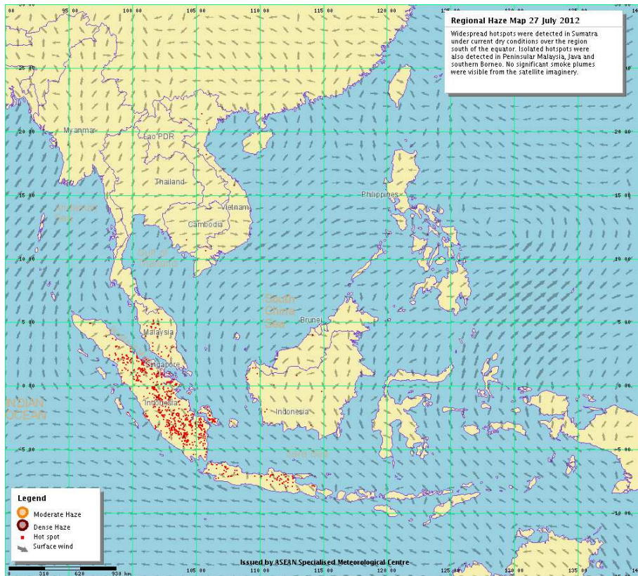
รูปที่ 2 ทิศทางลม เมื่อวันที่ 27 กรกฎาคม 2555
