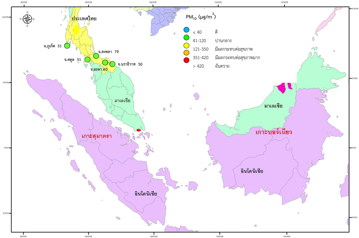
รูปที่ 3 แสดงค่าเฉลี่ยฝุ่นละอองขนาดไม่เกิน 10 ไมครอน ในเวลา 24 ชั่วโมง วันที่ 28 กรกฎาคม 2555
