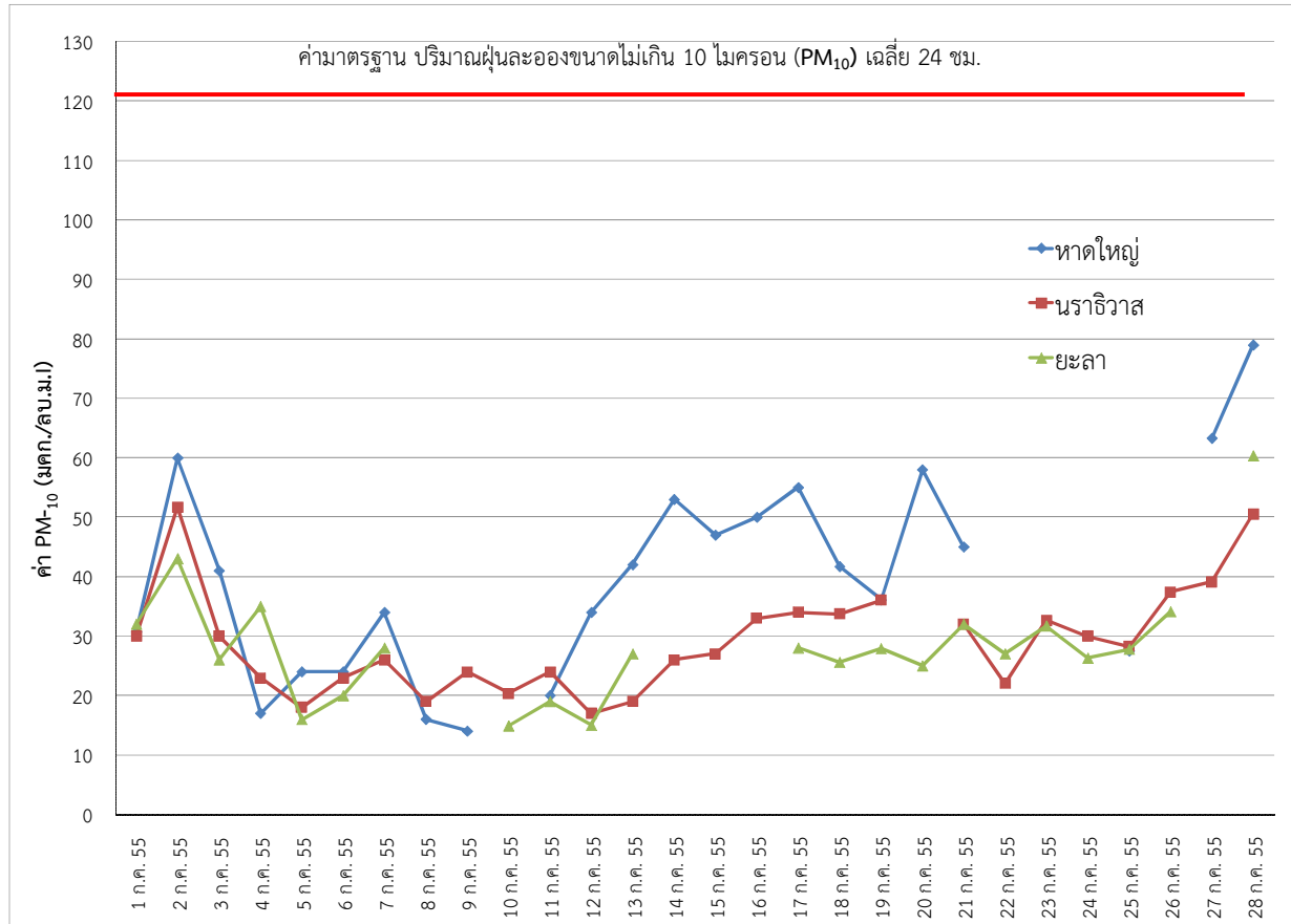
รูปที่ 5 แสดงการเปลี่ยนแปลงของปริมาณฝุ่นละอองขนาดไม่เกิน 10 ไมครอน (PM 10 ) ระหว่างวันที่ 1 - 28 กรกฎาคม 2555
