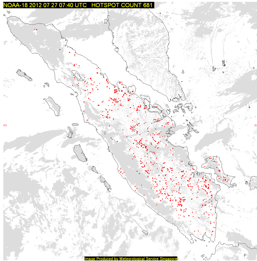
รูปที่ 1 จำนวนจุดที่เกิดไฟไหม้บนเกาะสุมาตรา ประเทศอินโดนีเซีย เมื่อวันที่ วันที่ 27 กรกฎาคม 2555
