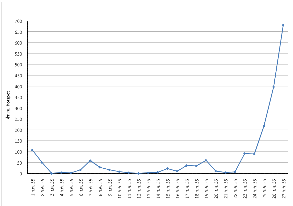
รูปที่ 4 แสดงการเปลี่ยนแปลงของจำนวน Hotspot บนเกาะสุมาตรา ระหว่างวันที่ 1 - 27 ก.ค. 2555
