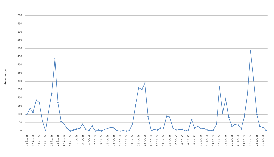
รูปที่ 4 แสดงการเปลี่ยนแปลงของ Hotspot บนเกาะสุมาตรา ระหว่างวันที่ 15 มิถุนายน - 31 สิงหาคม 2556
