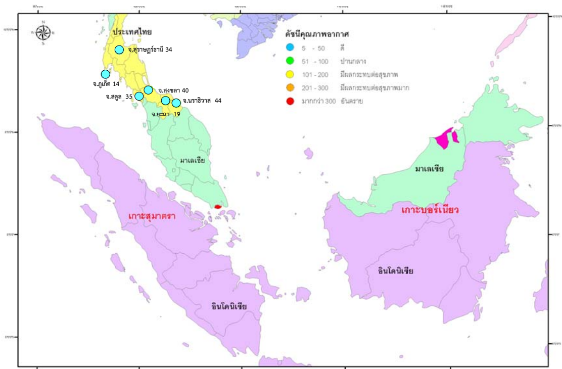
รูปที่ 3 ดัชนีคุณภาพอากาศ วันที่ 1 กันยายน 2556
