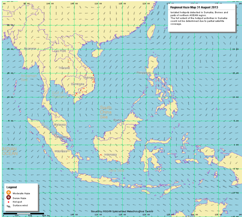
รูปที่ 2 ทิศทางลม เมื่อวันที่ 31 สิงหาคม 2556
