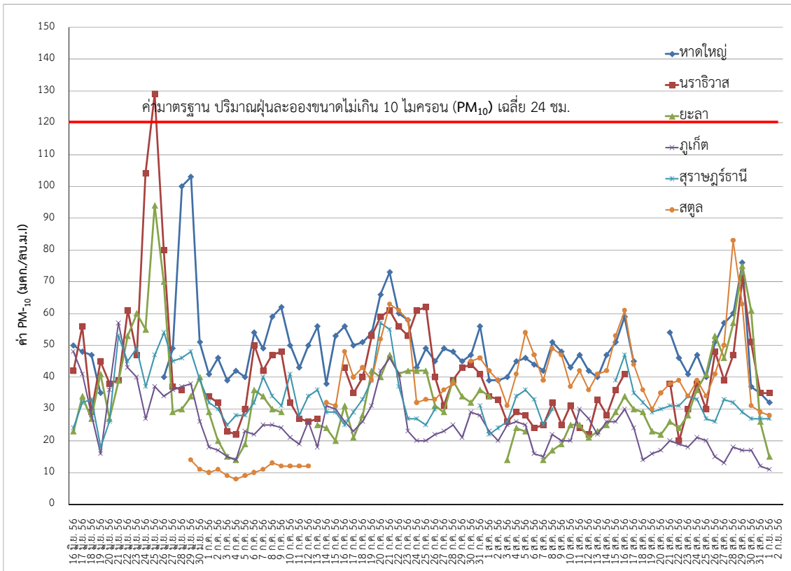
รูปที่ 5 แสดงการเปลี่ยนแปลงของปริมาณฝุ่นละอองขนาดไม่เกิน 10 ไมครอน (PM10) ระหว่างวันที่ 16 มิถุนายน - 1 กันยายน 2556
