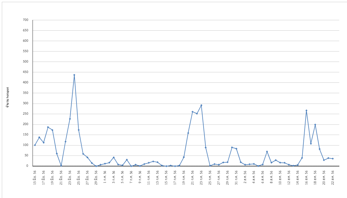
รูปที่ 4 แสดงการเปลี่ยนแปลงของ Hotspot บนเกาะสุมาตรา ระหว่างวันที่ 15 มิถุนายน - 22 สิงหาคม 2556
