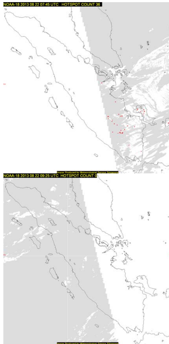
รูปที่ 1 จำนวนจุดที่เกิดไฟไหม้บนเกาะสุมาตรา เมื่อวันที่ 22 สิงหาคม 2556
