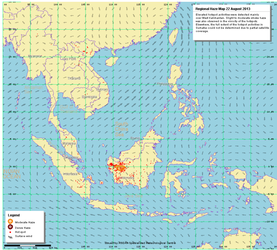
รูปที่ 2 ทิศทางลม เมื่อวันที่ 22 สิงหาคม 2556
