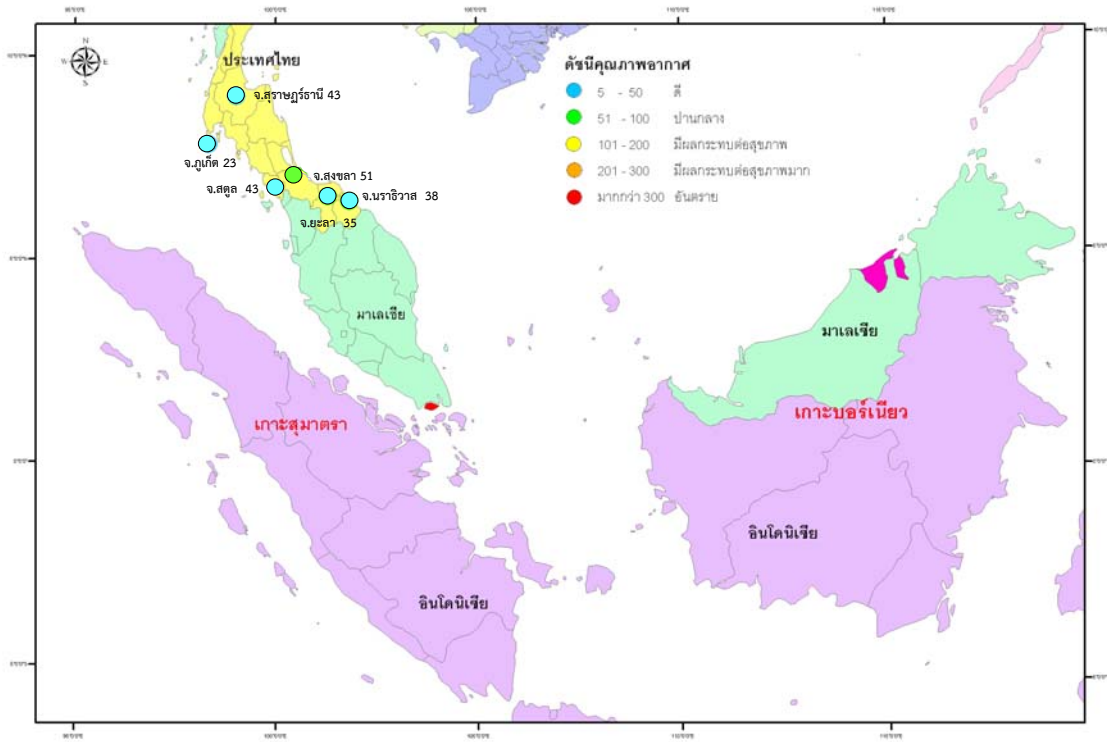
รูปที่ 3 ดัชนีคุณภาพอากาศ วันที่ 23 สิงหาคม 2556
