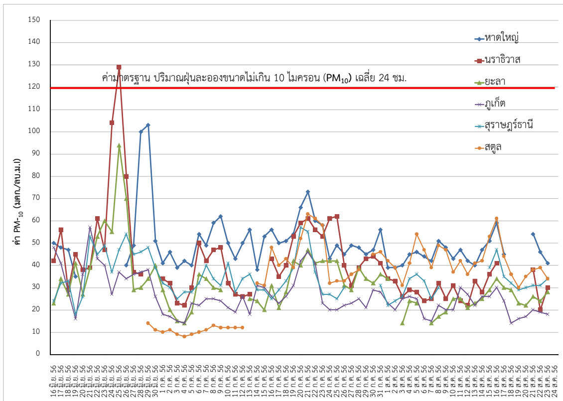
รูปที่ 5 แสดงการเปลี่ยนแปลงของปริมาณฝุ่นละอองขนาดไม่เกิน 10 ไมครอน (PM10) ระหว่างวันที่ 16 มิถุนายน - 23 สิงหาคม 2556
