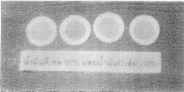
รูปที่ ข.2 กระดาษกรองวัดปริมาณควันทัวของน้ำมันดีเซล 90% ผสมน้ำมันปาล์ม 10%
