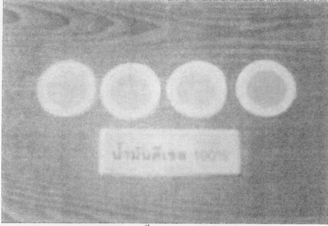
รูปที่ ข.1 กระดาษกรองวัดปริมาณควันทัวของน้ำมันดีเซล 100%
