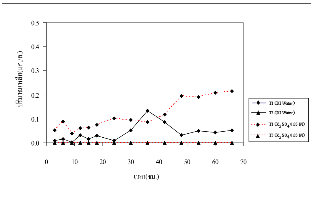
ภาพประกอบที่ 3-22 ปริมาณเหลือกับเวลาของ T1 และ T3 เมื่อถูกชะละลาย ด้วย deionized water และ K_2SO_4 0.05 โมล
