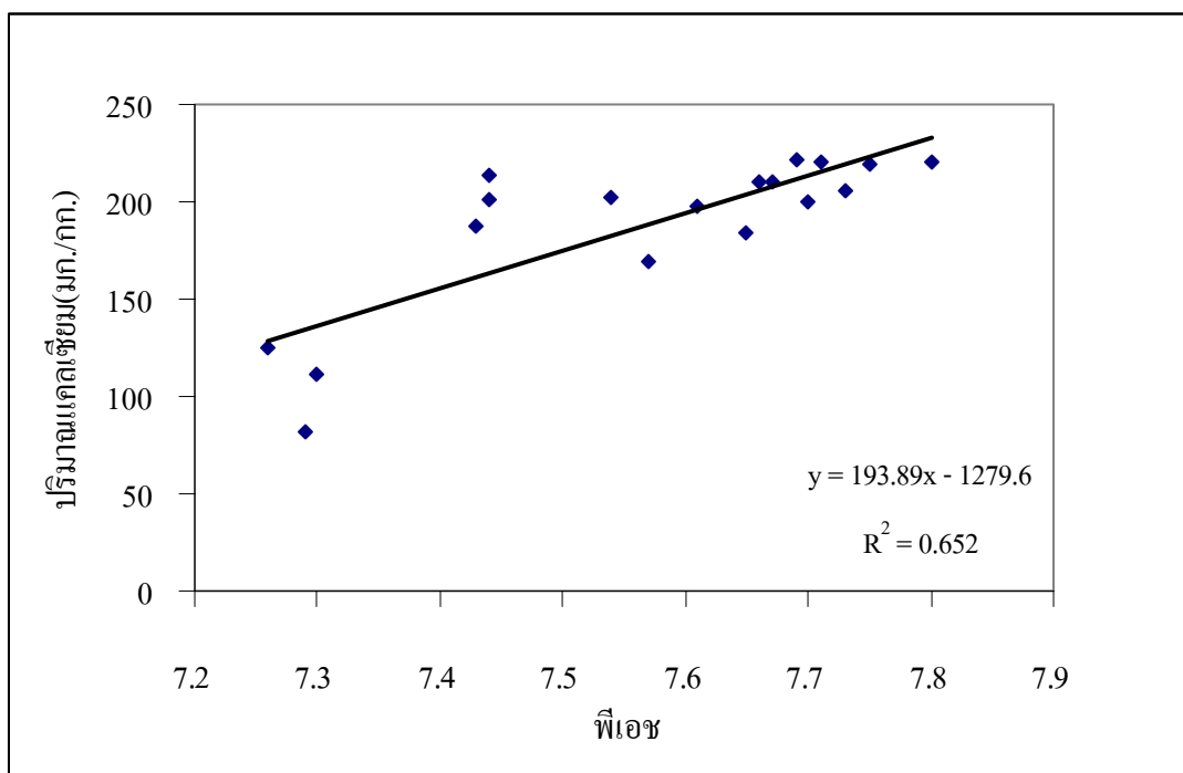
ภาพประกอบที่ 3-29 ความสัมพันธ์ระหว่างพีเอชกับปริมาณแคลเซียมในชุดการทดลองด้วยหินปูนฝุ่น
