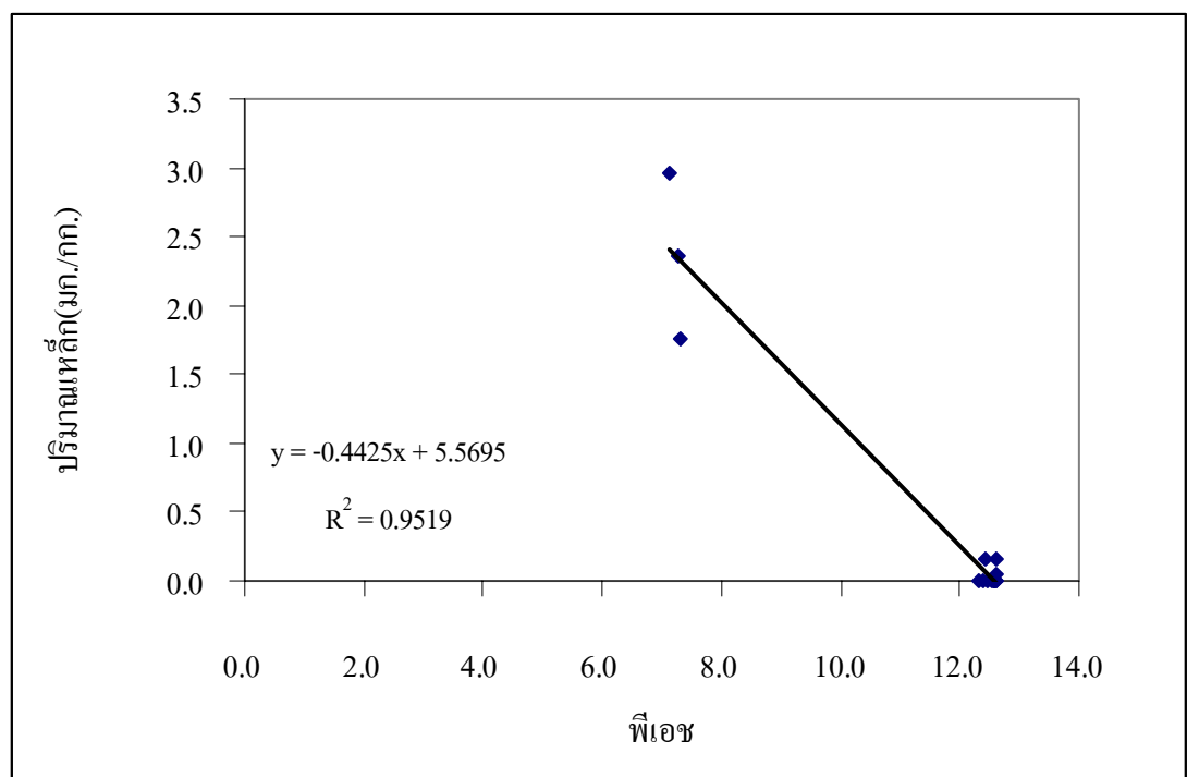
ภาพประกอบที่ 3-34 ความสัมพันธ์ระหว่างพีเอชกับปริมาณเหล็กในชุดการทดลองด้วยปูนขาว
