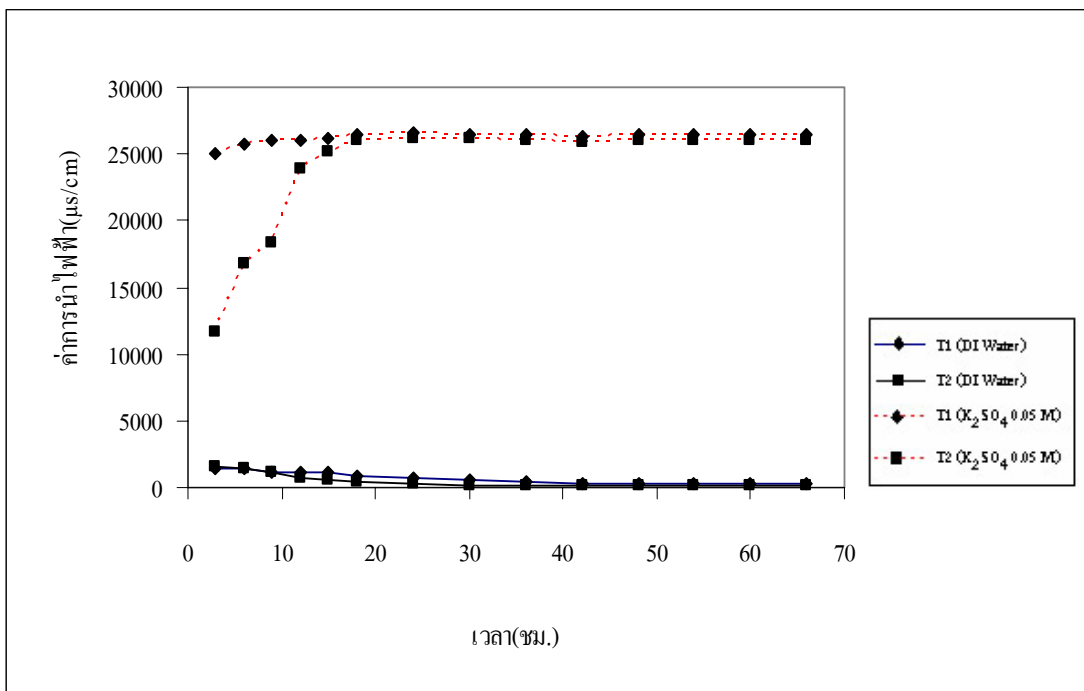
ภาพประกอบที่ 3-18 ค่าการนำไฟฟ้ากับเวลาของ T1 และ T2 เมื่อถูกชะละลายด้วย deionized water และ K 2 SO 4 0.05 โมล
