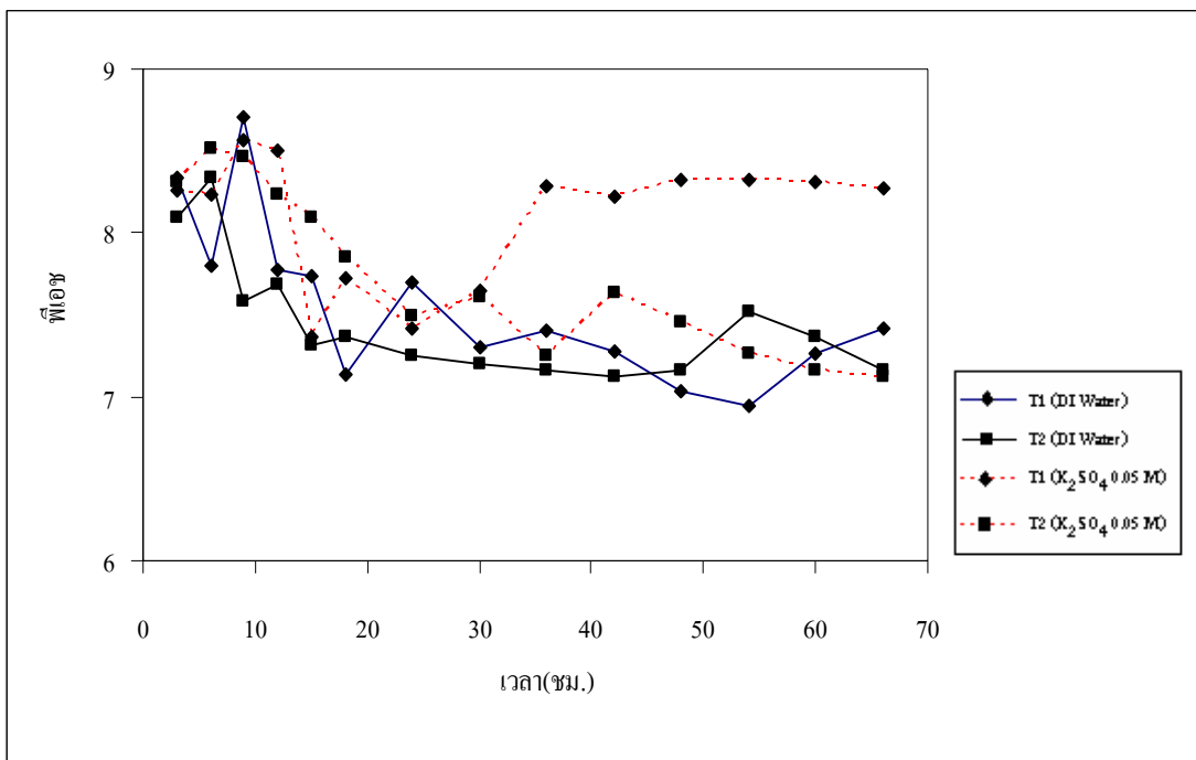
ภาพประกอบที่ 3-15 พีเอชกับเวลาของ T1 และ T2 เมื่อถูกระบายด้วย deionized water และ K_2SO_4 0.05 โมล
