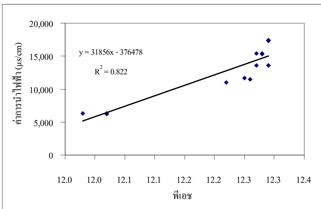
ภาพประกอบที่ 3-40 ความสัมพันธ์ระหว่างพีเอชกับค่าการนำไฟฟ้าในชุดการทดลองด้วยเถ้าลอย
