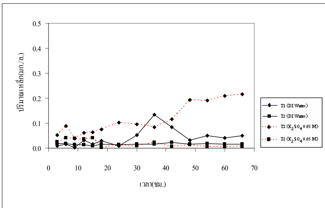
ภาพประกอบที่ 3-21 ปริมาณเหลือกับเวลาของ T1 และ T2 เมื่อถูกชะละลาย ด้วย deionized water และ K_2SO_4 0.05 โมล
