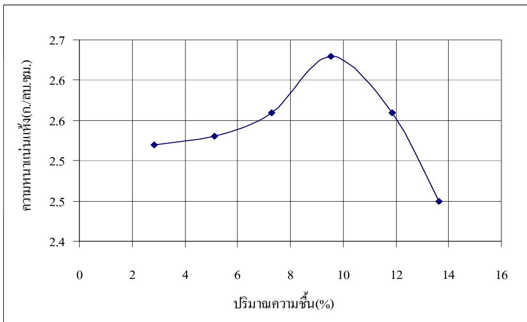
ภาพประกอบที่ 3-8 ความสัมพันธ์ระหว่างปริมาณน้ำ และความหนาแน่น ของชุดดินเหนืองแฉะ 100% w/w
