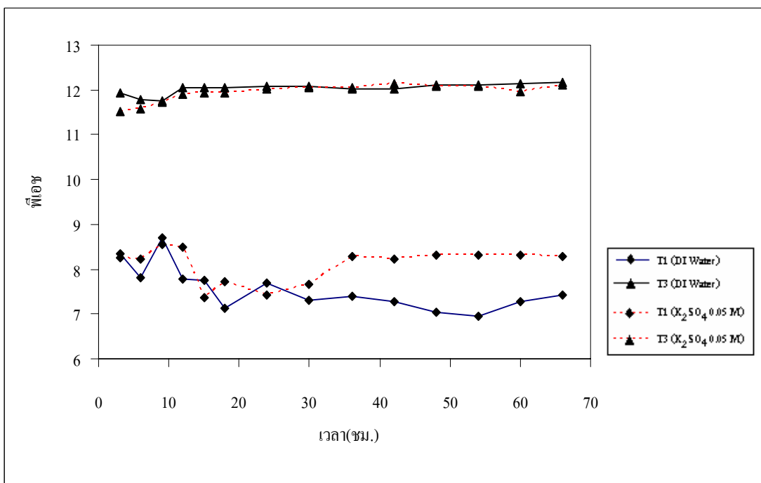
ภาพประกอบที่ 3-16 พีเอชกับเวลาของ T1 และ T3 เมื่อถูกระบายด้วย deionized water และ K_2SO_4 0.05 โมล
