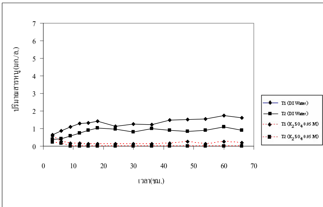
ภาพประกอบที่ 3-11 ปริมาณสารหนูกับเวลาของ T1 และ T2 เมื่อถูกชะละลาย ด้วย deionized water และ K 2 SO 4 0.05 โมล
