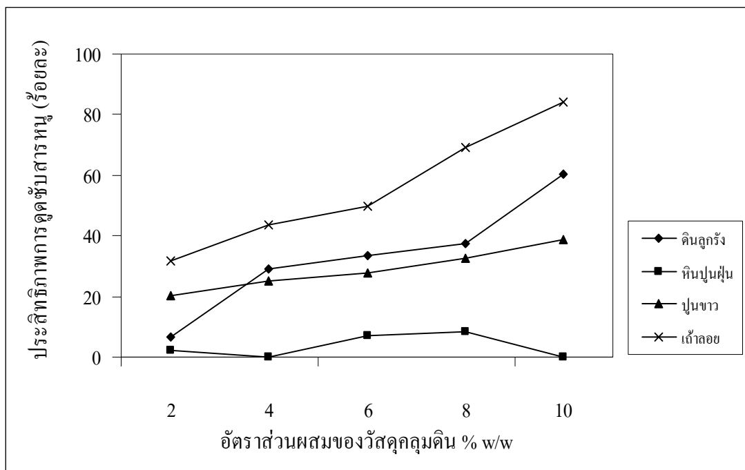
ภาพประกอบที่ 3-1 ประสิทธิภาพการดูดซับสารหนูโดยวัสดุคลุมดินทั้ง 4 ชนิด
