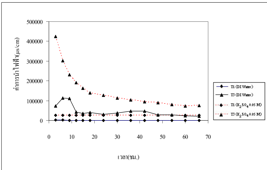
ภาพประกอบที่ 3-19 ค่าการนำไฟฟ้ากับเวลาของ T1 และ T3 เมื่อถูกชะละลายด้วย deionized water และ K 2 SO 4 0.05 โมล
