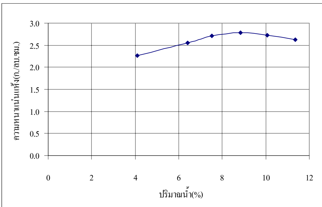
ภาพประกอบที่ 3-9 ความสัมพันธ์ระหว่างปริมาณน้ำ และความหนาแน่น ของชุดดินเหนืองแฉะผสมดินลูกรัง 20 % w/w
