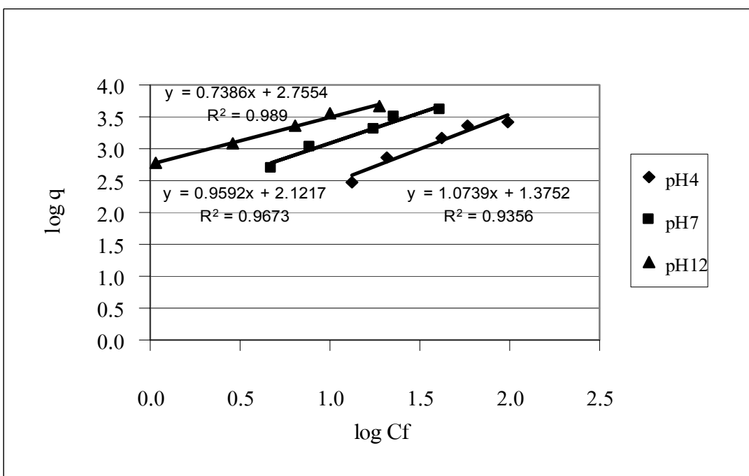
ภาพประกอบที่ 3-5 กราฟ Freundlich Isotherm ของเปลือกไข่
