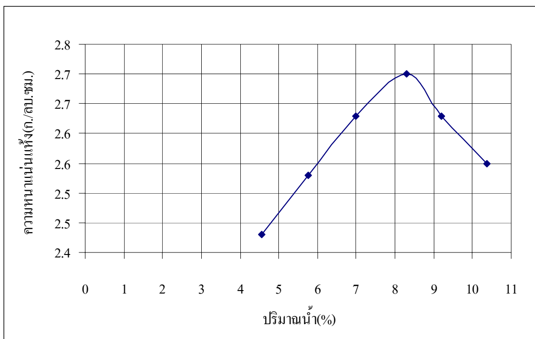
ภาพประกอบที่ 3-10 ความสัมพันธ์ระหว่างปริมาณน้ำ และความหนาแน่น ของชุดดินเหนืองแร่ผสมเถ้าลอย 10% w/w
