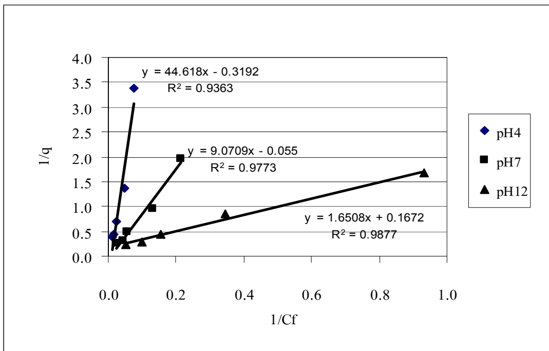
ภาพประกอบที่ 3-7 กราฟ Langmuir Isotherm ของน้ำ
