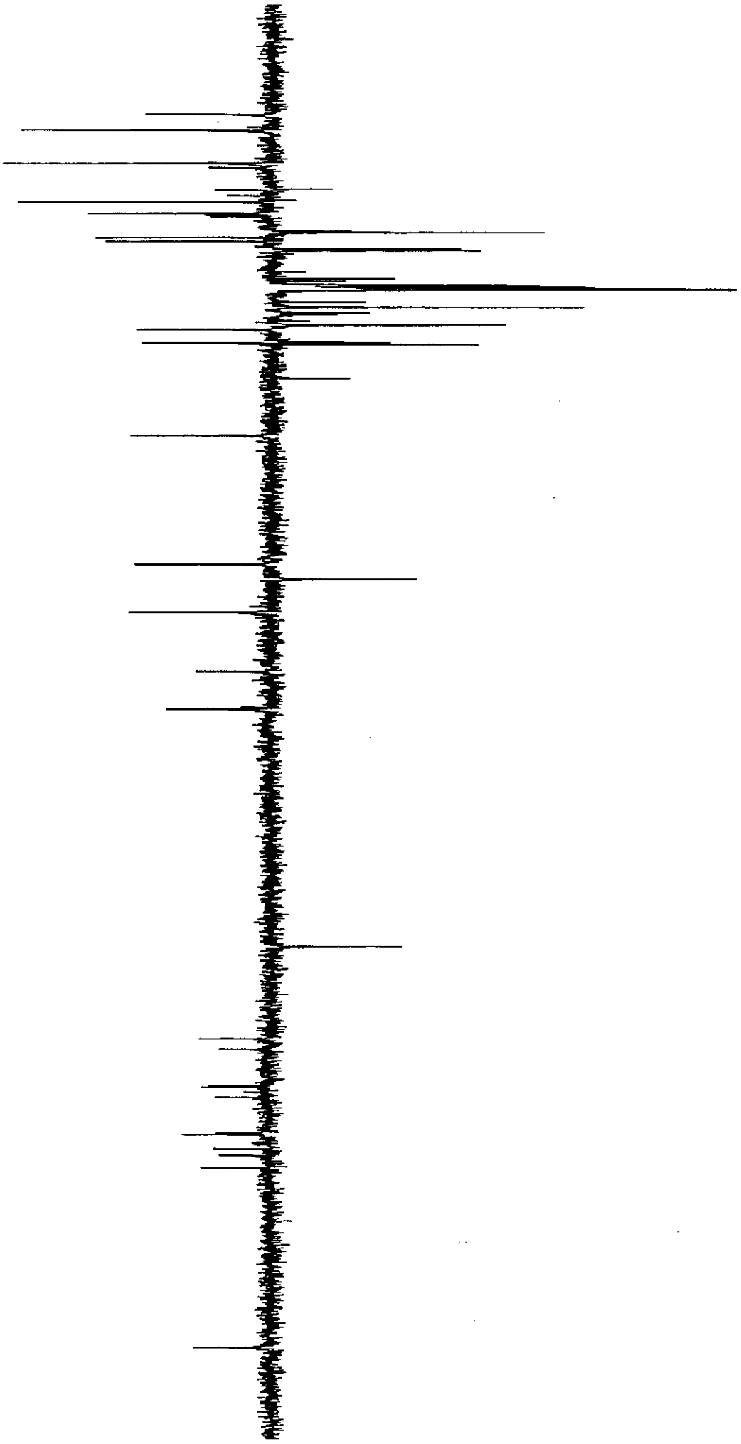
ภาพประกอบ 23 แสดง DEPT Spectrum ของสารผสม Excoecaria Factor I (3)
