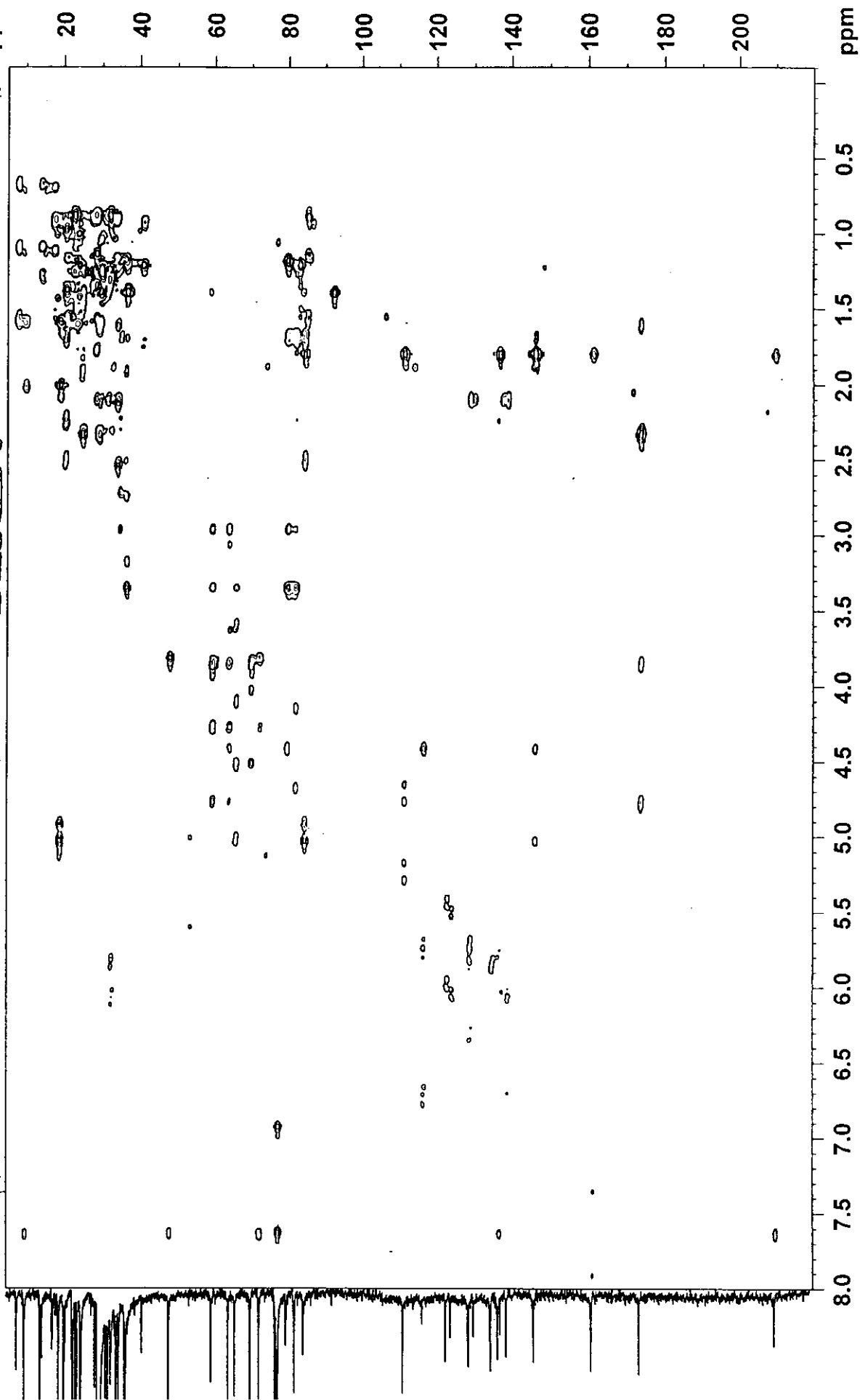
ภาพประกอบ 26 แสดง 2D HMBC Spectrum ของสารผสม Excoecaria Factor I (3)
