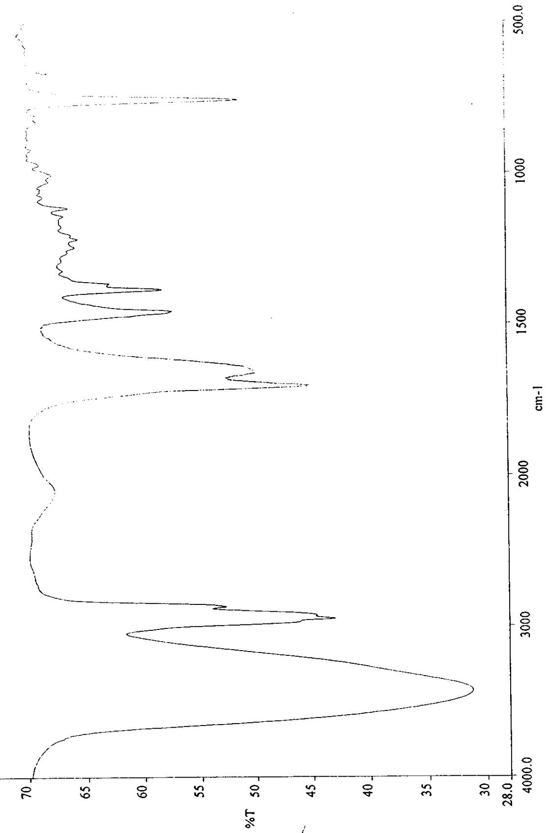
ภาพประกอบ 27 แสดง IR Spectrum (neat) ของสารผสม (4) และ (5)
