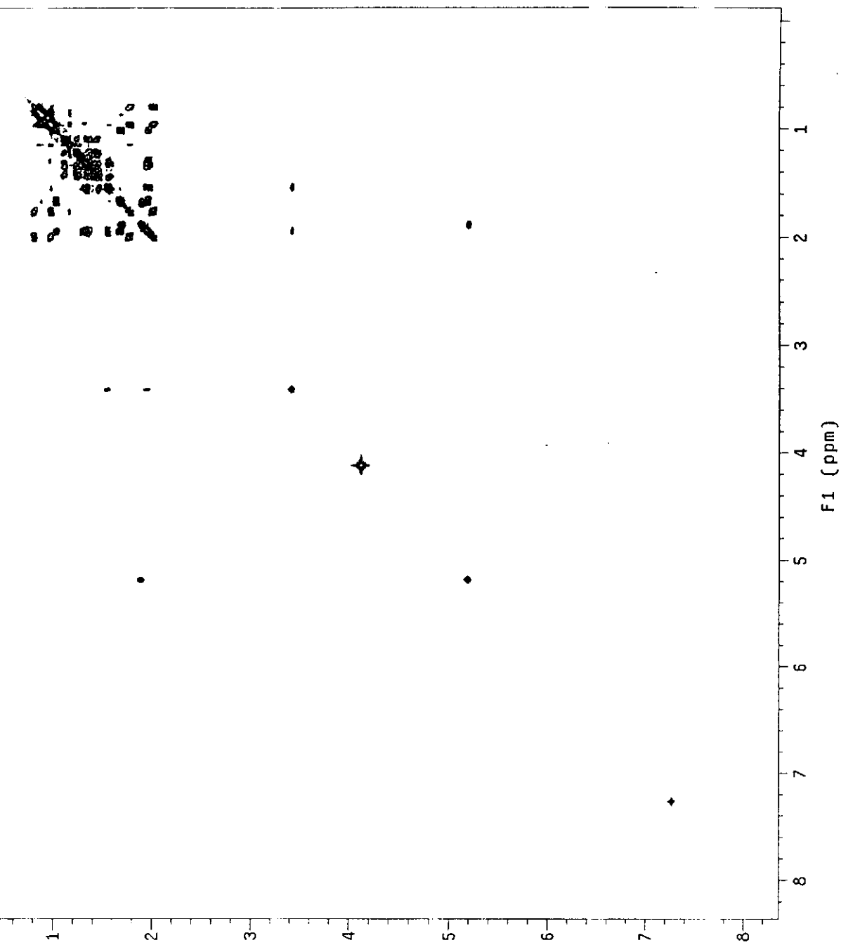
ภาพประกอบ 9 แสดง ^1\text{H} - ^1\text{H} COSY Spectrum ของสารประกอบ Olean-12-en-3 \alpha -ol (1)
