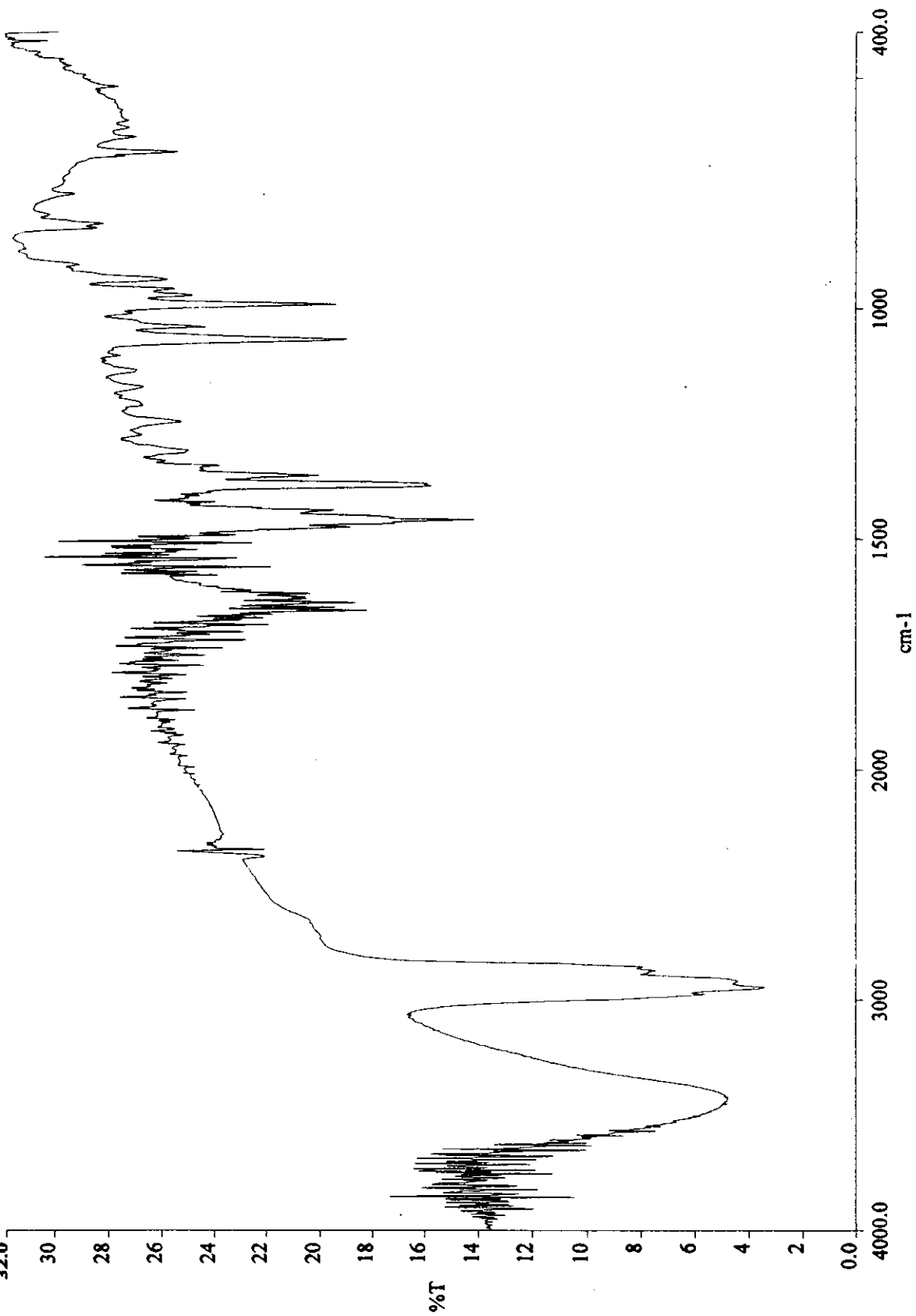
ภาพประกอบ 5 แสดง IR (KBr) Spectrum ของสารประกอบ Olean-12-en-3-ol (I)
