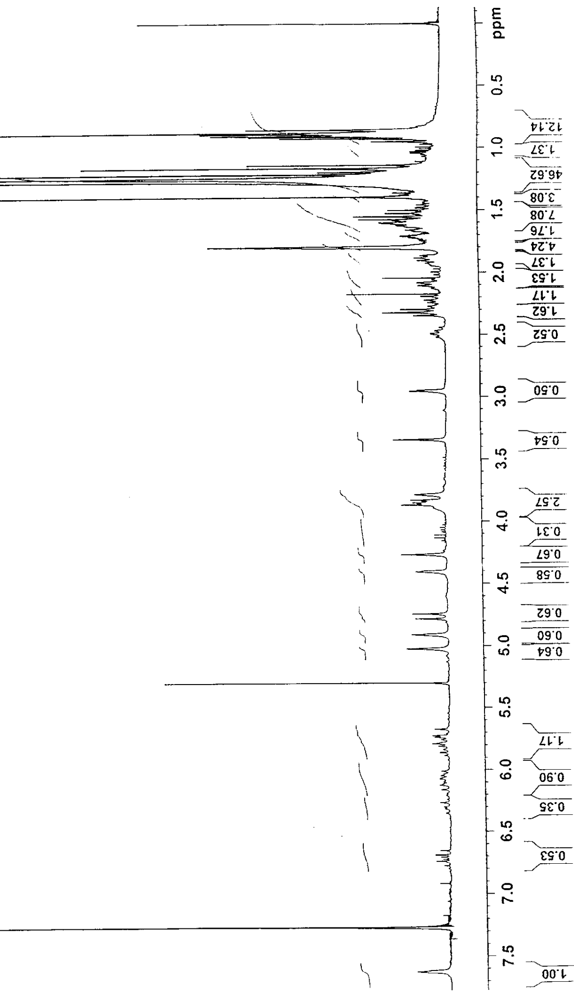
ภาพประกอบที่ 21 แสดง 1 H NMR Spectrum ( 300 MHz, CDCl 3 ) ของสารผสม Excoecaria Factor I (3)
