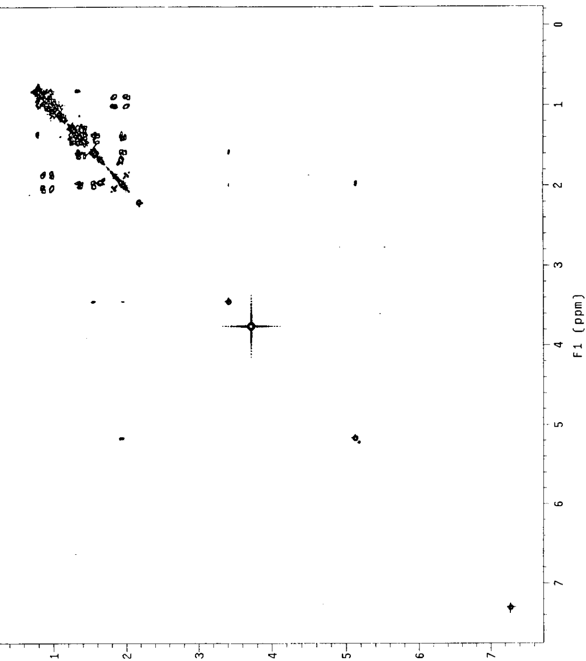
ภาพประกอบ 16 แสดง ^1\text{H} - ^1\text{H} COSY Spectrum ของสารประกอบ Urs-12-en-3-ol (2)
