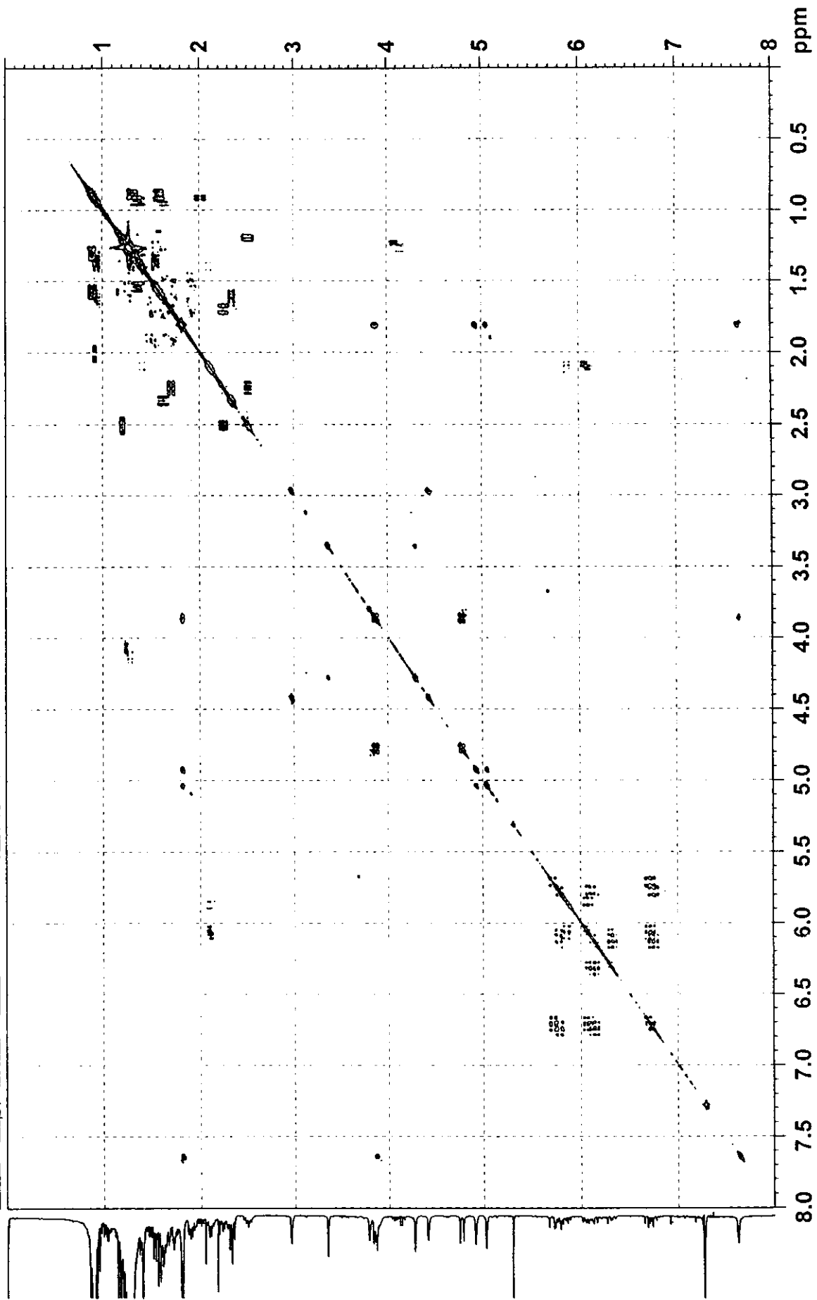
ภาพประกอบ 24 แสดง ^1\text{H} - ^1\text{H} COSY Spectrum ของสารผสม Excoecaria Factor I (3)
