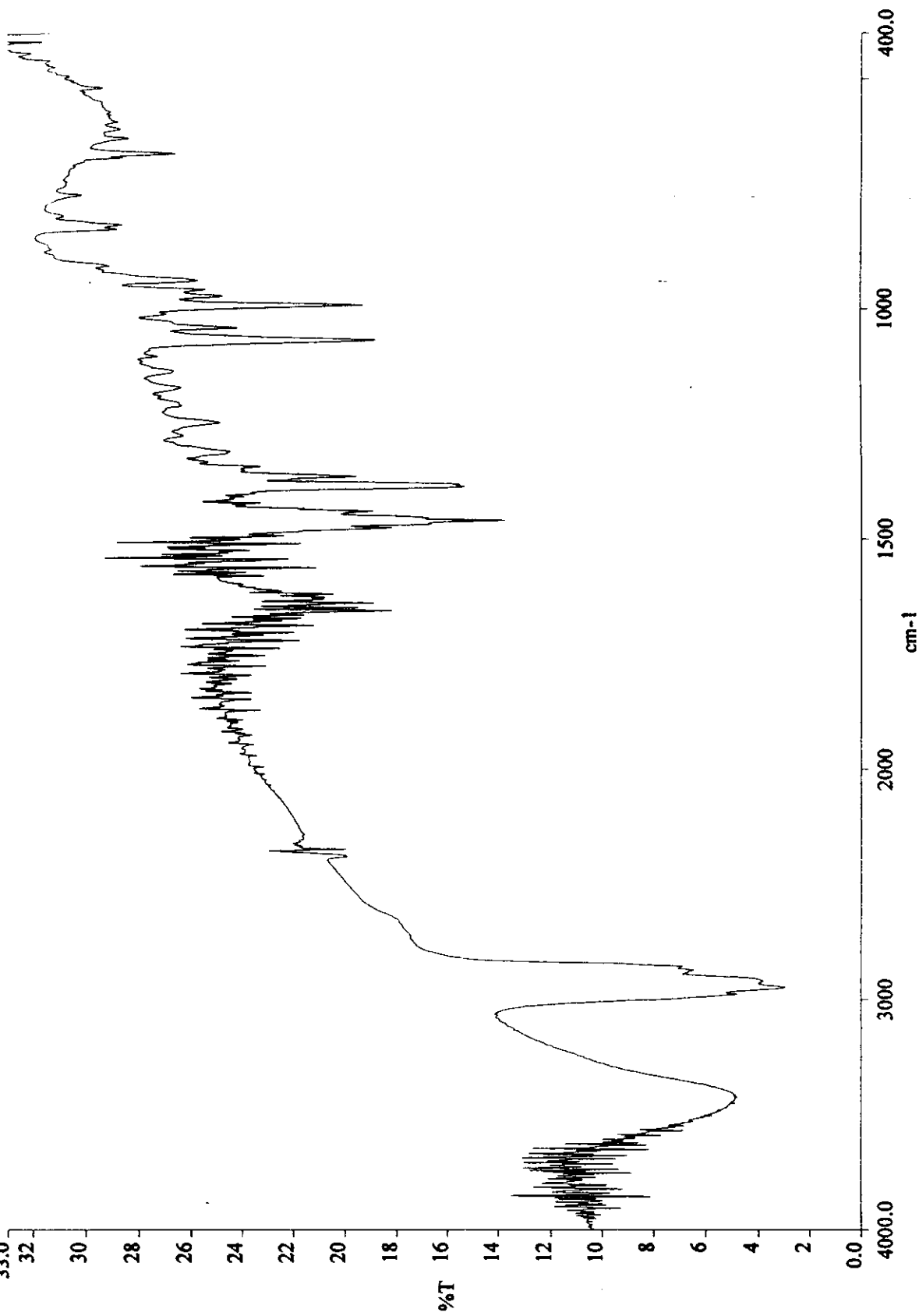
ภาพประกอบ 12 แสดง IR (KBr) Spectrum ของสารประกอบ Urs-12-en-3 \alpha -ol (2)
