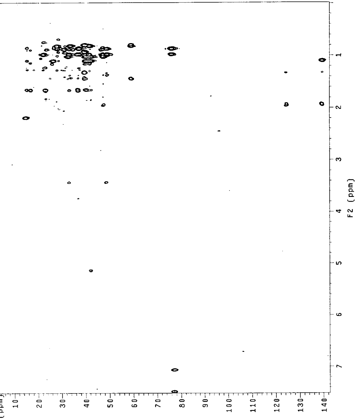
ภาพประกอบ 18 แสดง 2D HMBC Spectrum ของสารประกอบ Urs-12-en-3 \alpha -ol (2)
