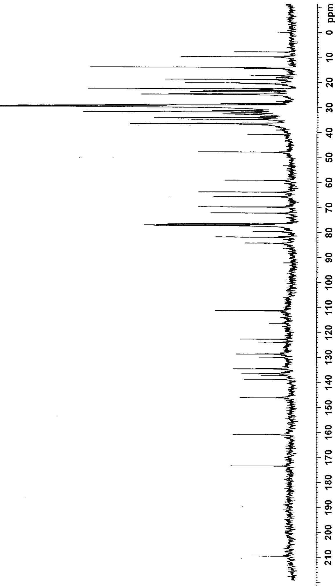
ภาพประกอบ 22 แสดง ^{13}\text{C} NMR Spectrum (100 MHz, \text{CDCl}_3 ) ของสารผสม Excoecaria Factor I (3)
