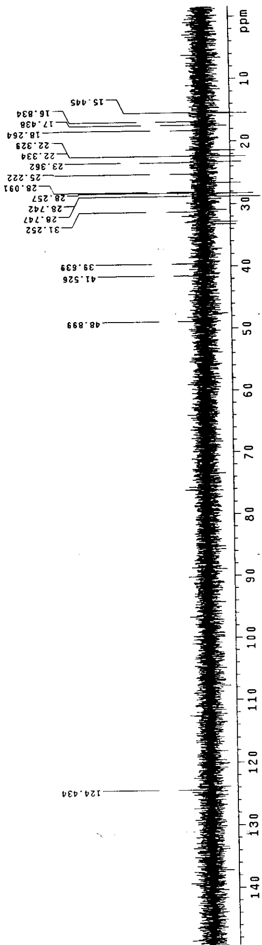
ภาพประกอบ 15 แสดง DEPT Spectrum ของสารประกอบ Urs-12-en-3 \alpha -ol (2)
