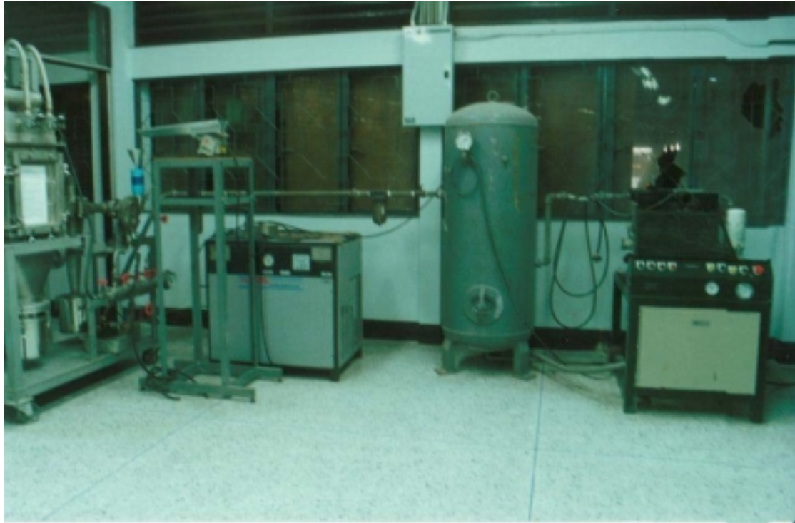
รูปผนวกที่ 3 ระบบโดยรวมของเครื่องบดละเอียดแบบ Jet mill
