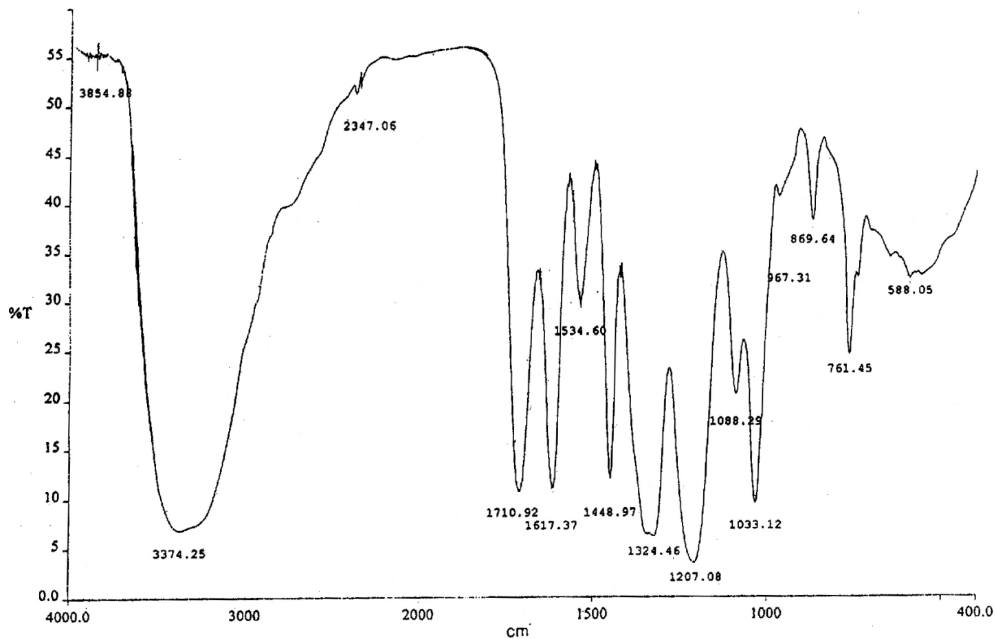
(D) Infrared spectrum of tannin
