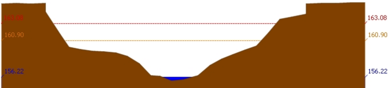
สถานี 120105T แม่น้ำป่าสักที่บ้านวังมเสหนือ ต.ทำอัญญ อ.หล่มสัก จ.เพชรบูรณ์ ระดับน้ำ 156.22 ม.รทก.
