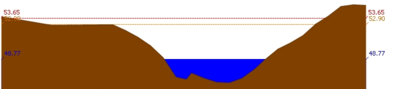
สถานี 120113T แม่น้ำป่าสักที่บ้านเขาค้าง ต.คลองกระจิง อ.ศรีเทพ จ.เพชรบูรณ์ ระดับน้ำ 48.77 ม.รทก.
