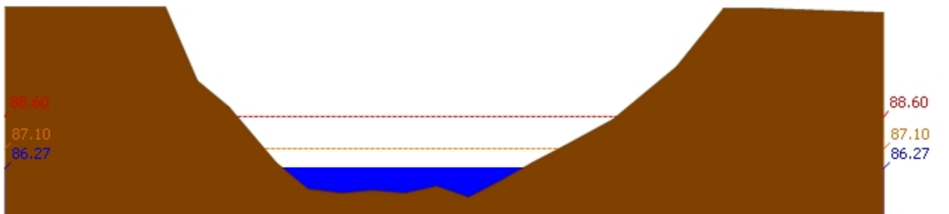
สถานี 120110T แม่น้ำป่าสักที่บ้านวังโบสถ์ ต.วังโบสถ์ อ.หนองไผ่ จ.เพชรบูรณ์ ระดับน้ำ 86.27 ม.รทก.
