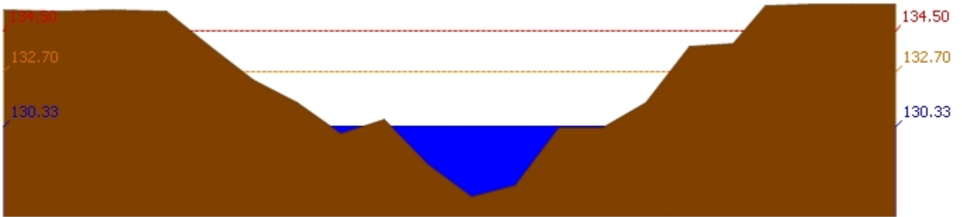
สถานี 120111T แม่น้ำป่าสักที่บ้านจางวาง ต.ลานบัว อ.หล่มสัก จ.เพชรบูรณ์ ระดับน้ำ 130.33 ม.รทก.
