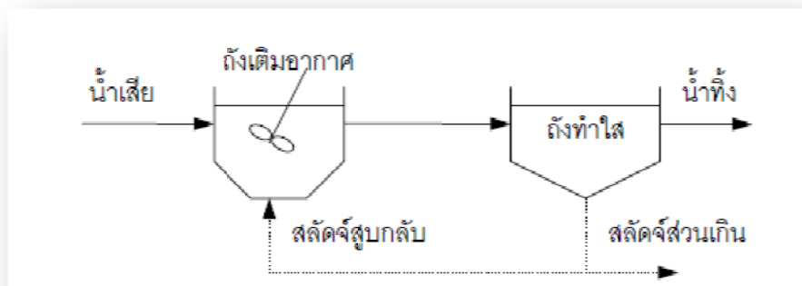
ตัวอย่าง แผนผังแสดงการทำงานของระบบบำบัดน้ำเสียสำหรับอาคาร
