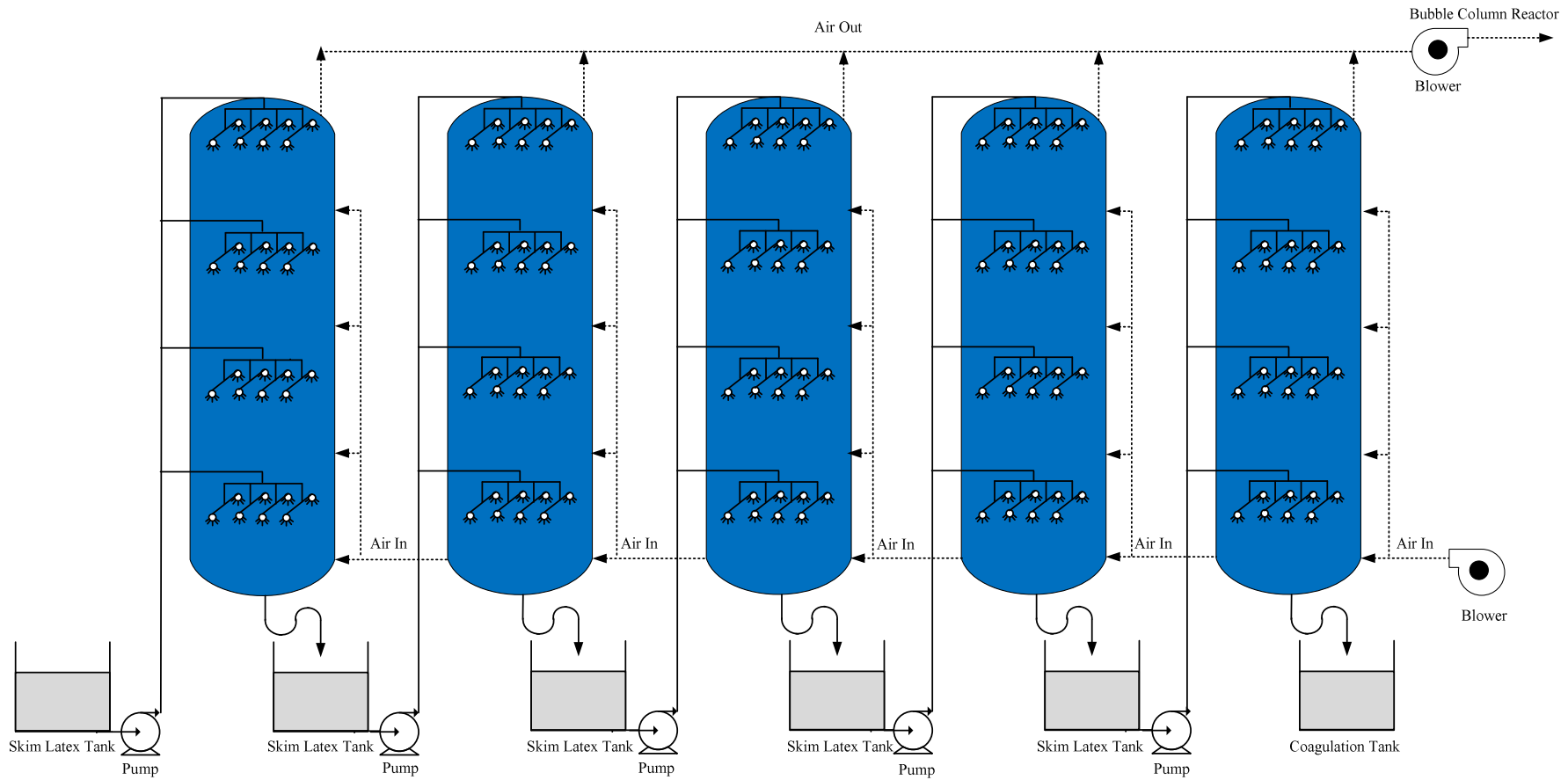
รูปที่ 4-22 ไดอะแกรมระบบคอลัมน์สเปรย์สำหรับใช้งานในโรงงานผลิตน้ำยางข้น
