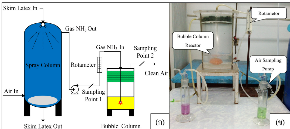
รูปที่ 3-15 ไดอะแกรมระบบปฏิกรณ์แก๊สแบบเปลขนาดต้นแบบสำหรับกำจัดแอมโมเนียในอากาศเสียจากระบบกำจัดแอมโมเนียในทางน้ำข้างด้วยคอลัมน์สเปรย์(ก) ระบบปฏิกรณ์แก๊สแบบเปลขนาดต้นแบบสำหรับกำจัดแอมโมเนียในอากาศเสียจากระบบกำจัดแอมโมเนียในทางน้ำข้างด้วยคอลัมน์สเปรย์ (ข)
