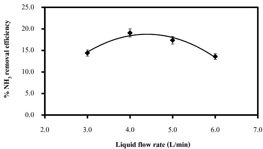
รูปที่ 4-3 ผลของอัตราการไหลของหางน้ำยางจำลองต่อประสิทธิภาพการกำจัดแอมโมเนียในหางน้ำยางจำลองด้วยระบบคอลัมน์สเปรย์ในเวลา 1 ชั่วโมง
