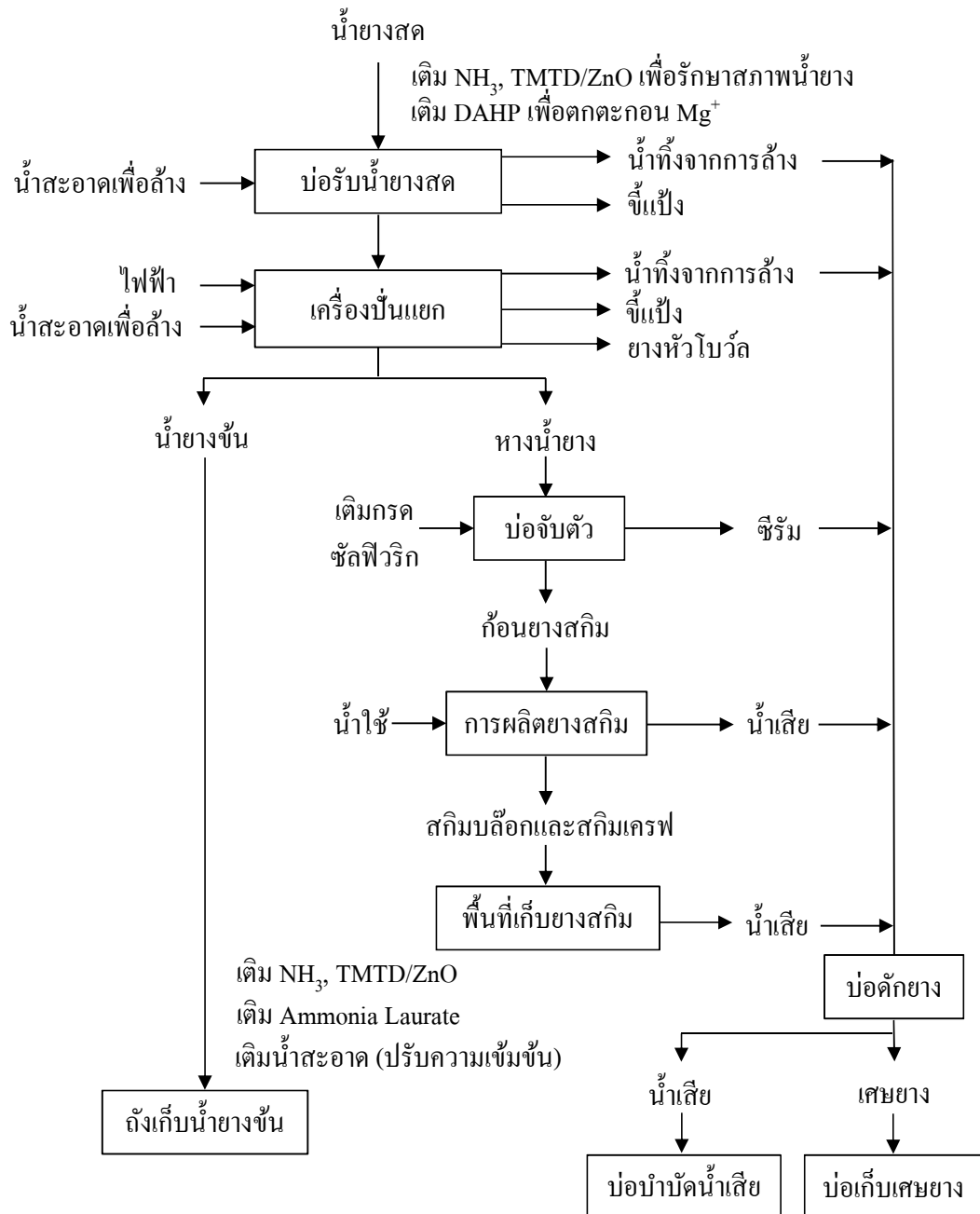
รูปที่ 2-1 กระบวนการผลิตน้ำยางข้นและหางน้ำยางด้วยกระบวนการปั่นแยก
