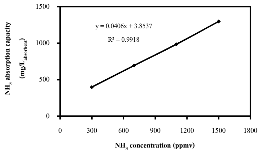
รูปที่ 4-16 ผลของความเข้มข้นแอมโมเนียในอากาศเสียจำลองต่อความสามารถในการดูดซึมแอมโมเนียของน้ำซีรั่มด้วยปฏิกรณ์แก๊สแบบเบิลขนาดห้องปฏิบัติการเป็นเวลา 7 ชั่วโมง
