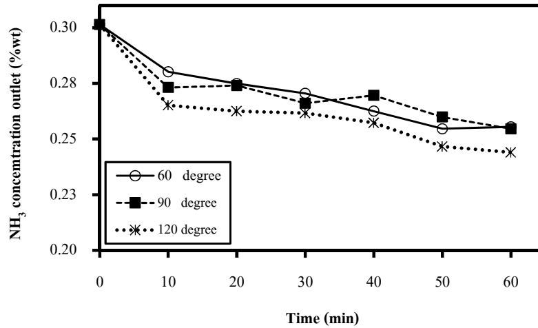
รูปที่ 4-1 ผลของมุมกระจายของหัวสเปรย์ต่อความเข้มข้นของแอมโมเนียในทางน้ำยางที่ทางออกของคอลัมน์สเปรย์กับเวลาที่ใช้ในการกำจัด
