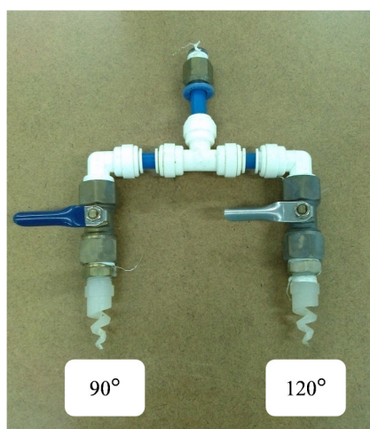
รูปที่ 4-5 การต่อหัวสเปรย์ 2 หัว แบบขนานระนาบเดียวกัน
