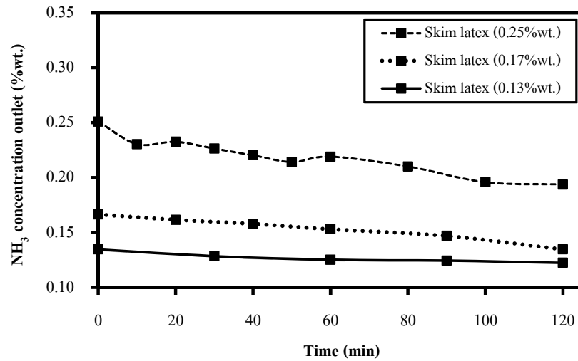
รูปที่ 4-10 ผลของหางน้ำยางจริงที่ระดับความเข้มข้นของแอมโมเนียต่างๆ ต่อความเข้มข้นของแอมโมเนียในหางน้ำยางทางออกของคอลัมน์สเปรย์กับเวลา
