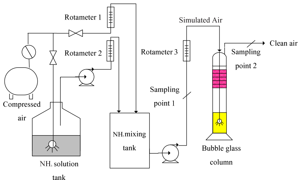
รูปที่ 3-13 ไดอะแกรมระบบปฏิกรณ์แก๊สแบบเบิลขนาดห้องปฏิบัติการสำหรับกำจัดแอมโมเนียในอากาศเสียจำลอง
