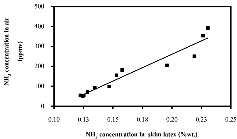
รูปที่ 4-13 ความเข้มข้นของแอมโมเนียในอากาศเสียที่ออกจากคอลัมน์สเปรย์สูง 1 เมตร กับความเข้มข้นของแอมโมเนียในหางน้ำยางจริง
