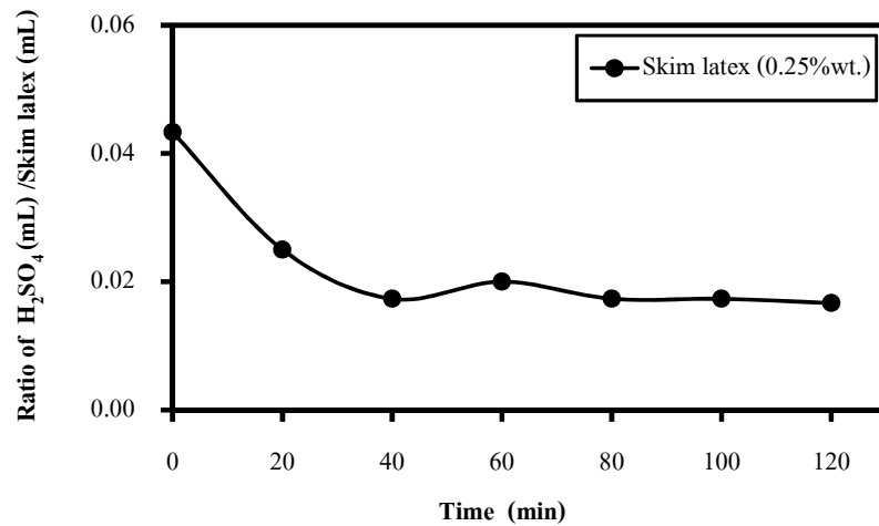
รูปที่ 4-11 สัดส่วนปริมาณการใช้กรดซัลฟูริกต่อปริมาณหางน้ำยางที่ใช้จับตัวเนื้อยางสกินที่เวลาต่างๆ ในการกำจัดแอมโมเนียในหางน้ำยางด้วยคอลัมน์สเปรย์
