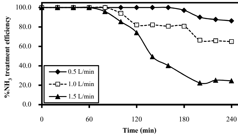
รูปที่ 4-17 ผลของอัตราการไหลของอากาศเสียจำลองต่อประสิทธิภาพการกำจัดแอมโมเนียด้วย ปฏิกรณ์แก๊สแบบเปิดขนาดห้องปฏิบัติการกับเวลาโดยการใช้ น้ำชีวมเป็น สารดูดซับที่ระดับความเข้มข้นของแอมโมเนียในอากาศเสียจำลอง 1,100 ppmv
