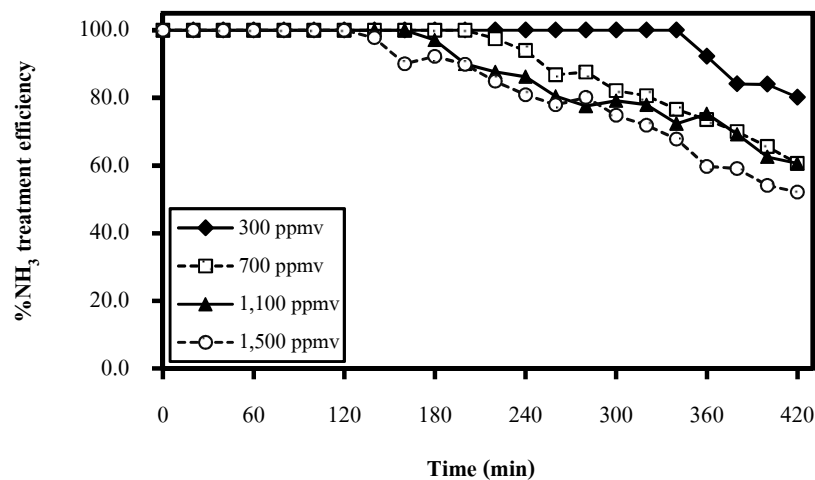
รูปที่ 4-15 ผลของความเข้มข้นของแอมโมเนียในอากาศเสียจำลองต่อประสิทธิภาพการกำจัดแอมโมเนียกับเวลาด้วยปฏิกรณ์แก๊สแบบเบิลขนาดห้องปฏิบัติการ โดยใช้น้ำซีรัม
