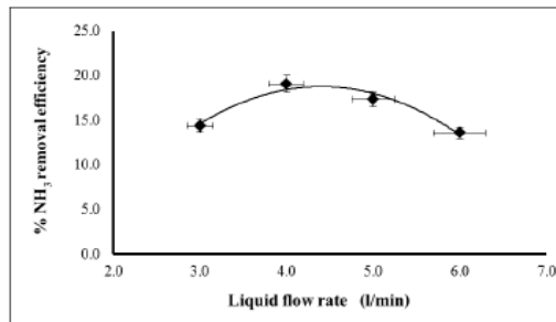
รูปที่ 4 แสดงผลของอัตราการไหลของเหลวต่อประสิทธิภาพการกำจัดแอมโมเนียในหาน้ำอย่างจำลองที่เวลา 1 ชั่วโมง
