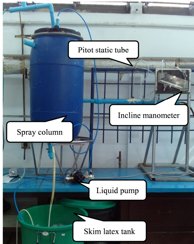
รูปที่ 3-4 ระบบคอลัมน์สเปรย์สำหรับกำจัดแอมโมเนียในทางน้ำยาง
