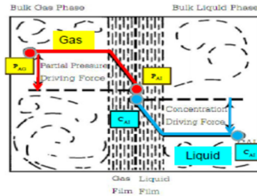
รูปที่ 2-3 ทฤษฎีเยื่อ 2 ชั้น
