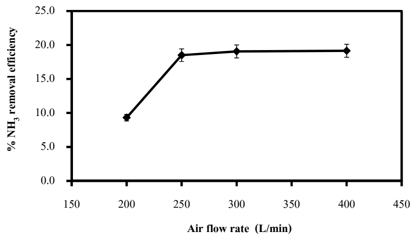
รูปที่ 4-2 ประสิทธิภาพการกำจัดแอมโมเนียในทางน้ำยางจำลองด้วยระบบคอลัมน์สเปรย์ที่อัตราการไหลของอากาศต่างๆในเวลา 1 ชั่วโมง
