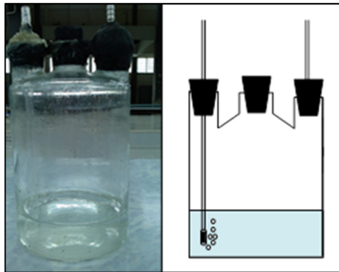
รูปที่ 3-12 ขวดบรรจุแอมโมเนียมไฮดรอกไซด์เพื่อผลิตอากาศเสียจำลองที่มีแก๊สแอมโมเนีย ปนเปื้อน
