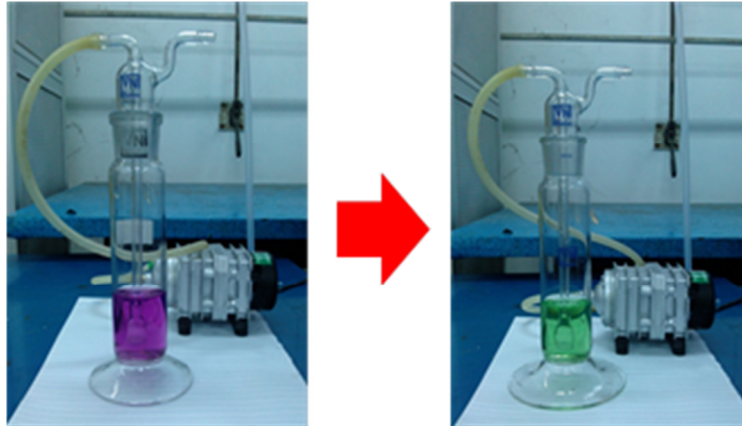
รูปที่ 3-20 การเก็บตัวอย่างแอมโมเนียในอากาศเสียด้วยอิมพิงเจอร์
