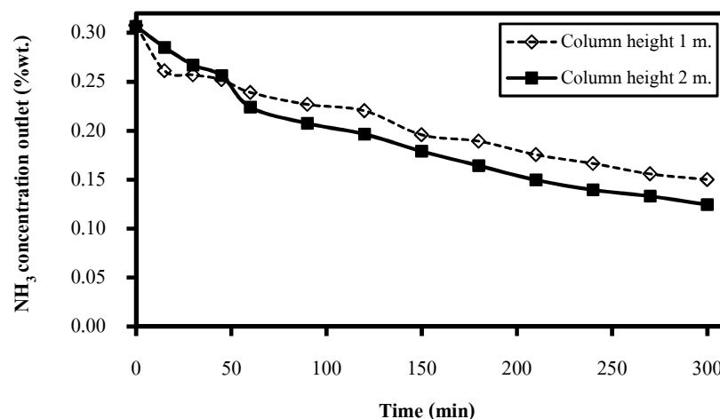
รูปที่ 4-4 ผลของความสูงของคอลัมน์สเปรย์ต่อความเข้มข้นของแอมโมเนียในหางน้ำยางจำลองที่ทางออกของคอลัมน์สเปรย์กับเวลาในการดำเนินการทดลอง
