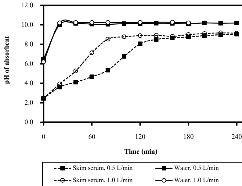
รูปที่ 4-20 การเปลี่ยนแปลงค่า pH ในระหว่างการดูดซึมแก๊สแอมโมเนียที่ปนเปื้อนในอากาศเสียจำลองกับเวลา ที่ระดับความเข้มข้นของแอมโมเนีย 1,100 ppmv ในเวลา 4 ชั่วโมง
