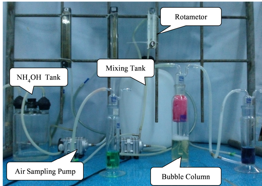
รูปที่ 3-14 ระบบปฏิบัติการแก๊สบำบัดขนาดห้องปฏิบัติการสำหรับกำจัด แอมโมเนียในอากาศเสียจำลอง
