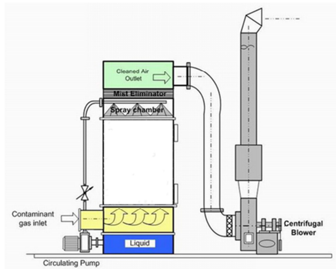
รูปที่ 2-4 คอลัมน์สเปรย์
