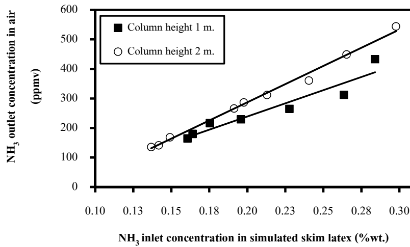
รูปที่ 4-12 ความเข้มข้นของแอมโมเนียในอากาศเสียจากคอลัมน์สเปรย์ที่มีความสูงต่างๆ กับความเข้มข้นของแอมโมเนียในหางน้ำยางจำลอง
