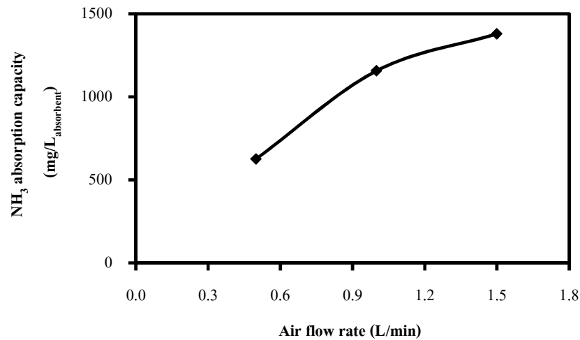
รูปที่ 4-18 ผลของอัตราการไหลของแอมโมเนียในอากาศเสียจำลองต่อความสามารถในการดูดซึมแอมโมเนียของน้ำซีรัมด้วยปฏิกรณ์แก๊สแบบเบิลขนาดห้องปฏิบัติการที่ระดับความเข้มข้นของแอมโมเนีย 1,100 ppmv ในเวลา 4 ชั่วโมง
