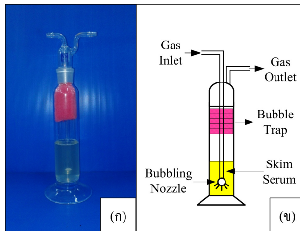
รูปที่ 3-8 ปฏิกรณ์แก๊สبابเบิลขนาดห้องปฏิบัติการสำหรับกำจัดแอมโมเนียในอากาศเสียจำลอง (ก) และไดอะแกรมปฏิกรณ์แก๊สبابเบิลขนาดห้องปฏิบัติการสำหรับกำจัดแอมโมเนียในอากาศเสียจำลอง (ข)
