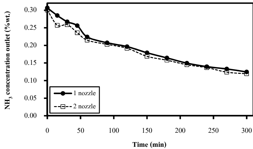
รูปที่ 4-9 ผลจำนวนหัวหัวสเปรย์ต่อความเข้มข้นของแอมโมเนียในหางน้ำยางจำลองที่ทางออกของคอลัมน์สเปรย์สูง 2 เมตร กับเวลาในการทดลอง
