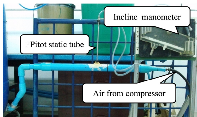
รูปที่ 3-7 ระบบการวัดอัตราการไหลของกระแสอากาศป้อนของคอลัมน์สเปรย์
