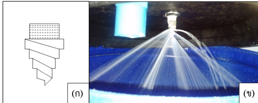
รูปที่ 3-6 ไดอะแกรมของหัวสเปรย์ชนิดเกลียวเดียวหมุน (ก) และลักษณะการติดตั้งหัวสเปรย์ (ข)
