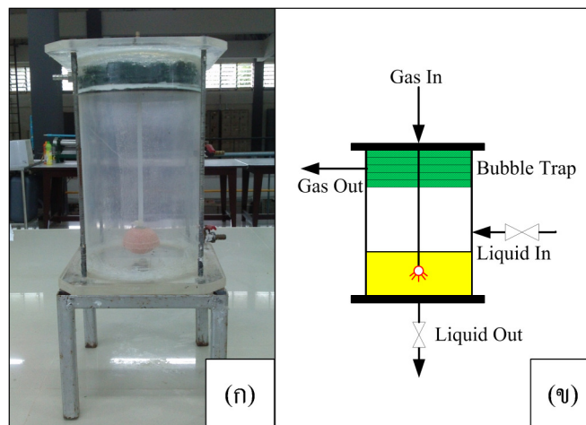
รูปที่ 3-9 ปฏิกรณ์แก๊สแบบเบิลขนาดต้นแบบสำหรับกำจัดแอมโมเนียในอากาศเสียจากระบบคอลัมน์สเปรย์ (ก) และไดอะแกรมปฏิกรณ์แก๊สแบบเบิลขนาดต้นแบบสำหรับกำจัดแอมโมเนียในอากาศเสียจากระบบคอลัมน์สเปรย์ (ข)
