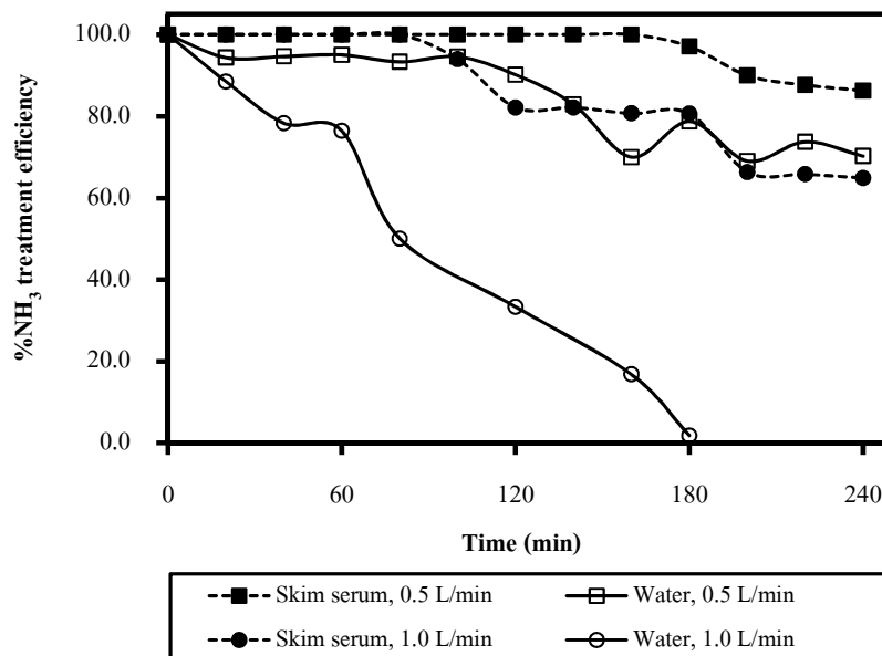
รูปที่ 4-19 การเปรียบเทียบประสิทธิภาพการกำจัดแอมโมเนียที่ปนเปื้อนในอากาศเสียจำลองกับเวลา โดยการใช้น้ำชีรั่มและน้ำเป็นสารดูดซับ ที่ระดับความเข้มข้นของแอมโมเนีย ในอากาศเสียจำลอง 1,100 ppmv
