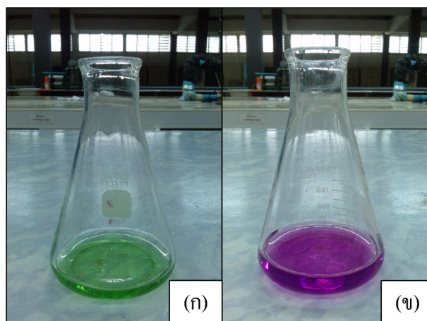
รูปที่ 3-18 สีของสารละลายก่อน (ก) และหลัง (ข) การไทเทรตหางน้ำยางจำลอง
