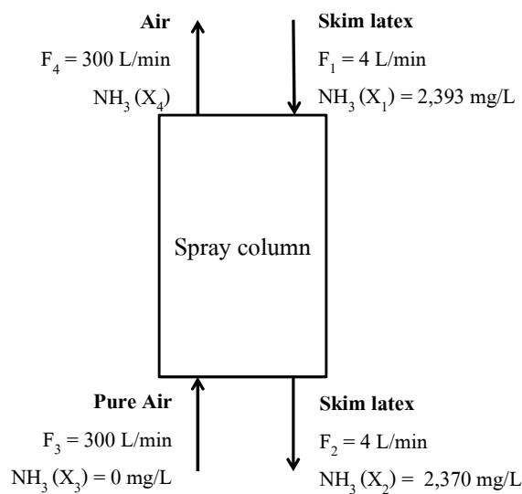
รูปที่ 4-14 การดุลมวลของแอมโมเนียในระบบคอลัมน์สเปรย์
