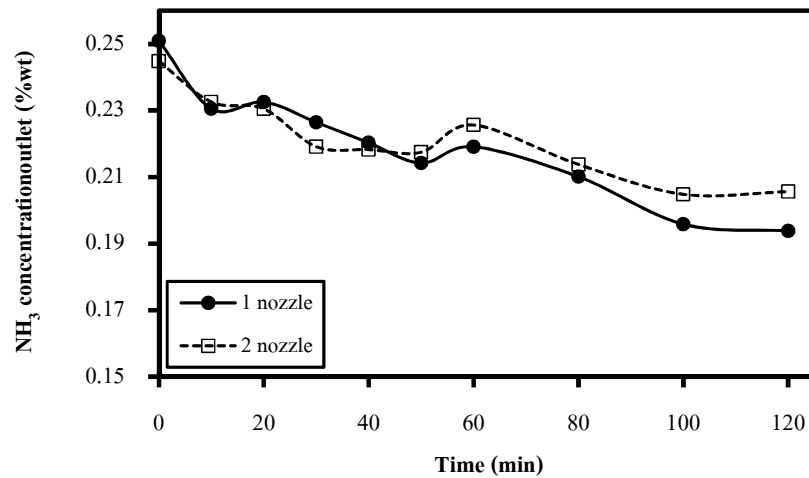
รูปที่ 4-6 ผลจำนวนหัวหัวสเปรย์ต่อความเข้มข้นของแอมโมเนียในทางน้ำยางที่ทางออกของคอลัมน์สเปรย์กับเวลาในการทดลอง
