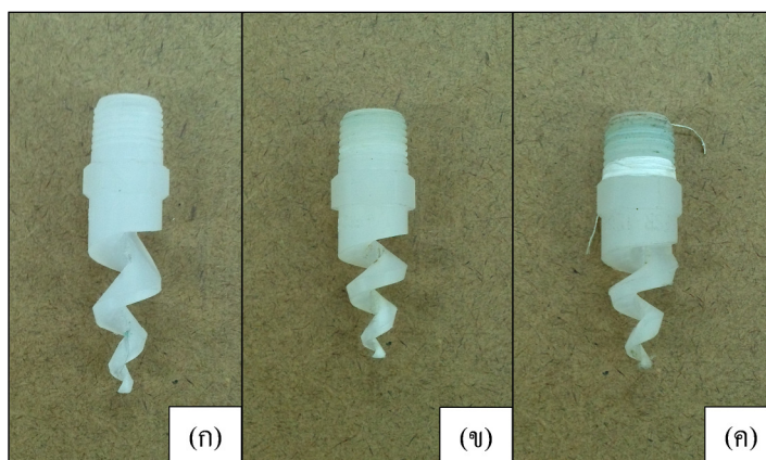
รูปที่ 3-10 หัวสเปร์ยชนิดเกลียวเดียวมุมกระจายตัว 60°(ก) 90°(ข) และ 120°(ค)
