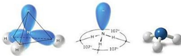
รูปที่ 2-2 รูปร่างโมเลกุลของแอมโมเนีย
