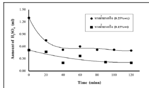
รูปที่ 8 แสดงผลปริมาณการใช้กรดซัลฟูริก 98% ในการจับตัวเนื้อยางที่เวลาต่างๆ
