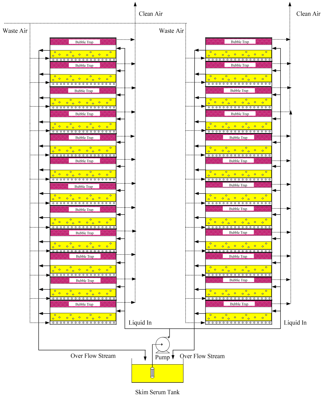
รูปที่ 4-23 ไคอะแกรมระบบปฏิบัติการแก๊สบำบัดสำหรับกำจัดแอมโมเนียในอากาศเสียจากคอกหมู สเปรย์
