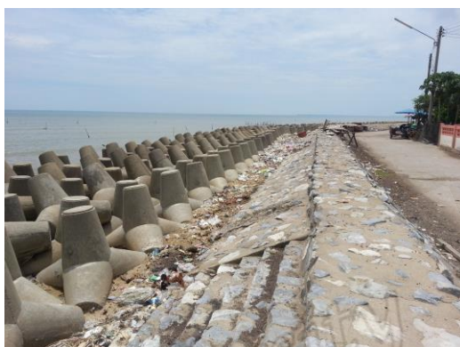
“ตุ๊กตาญี่ปุ่น” ใช้เป็นแนวป้องกันการกัดเซาะชายฝั่ง
