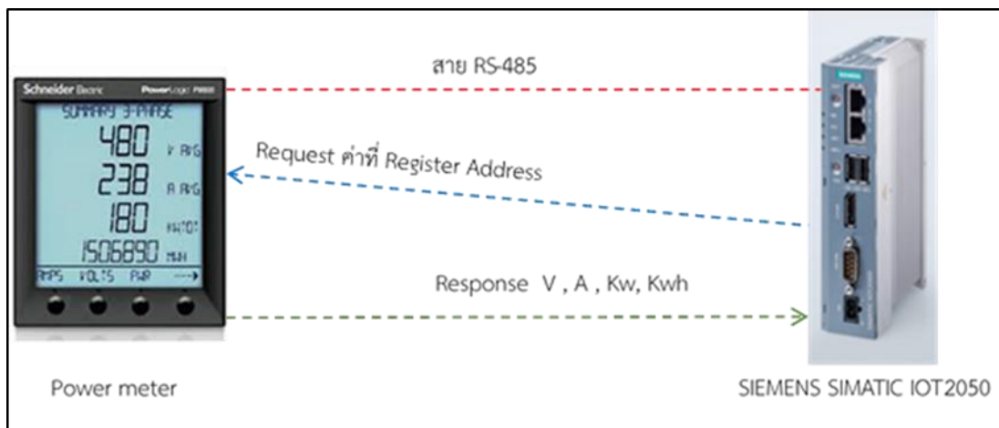
ภาพที่ 22 การเชื่อมต่ออุปกรณ์ Multi-Function Digital Power Meter กับ SIEMENS SIMATIC IOT2050 ผ่านทางพอร์ต Serial RS-485 Protocol Modbus RTU
