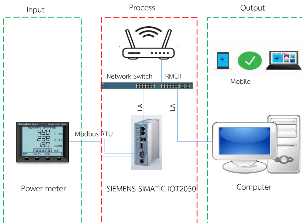
ภาพที่ 16 การออกแบบฮาร์ดแวร์และการเชื่อมต่อกับอุปกรณ์ SIEMENS SIMATIC IOT2050
