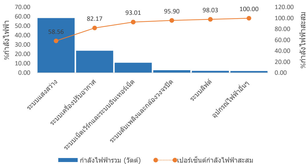
ภาพที่ 52 แผนภูมิพาเรโต (Pareto Diagram)
