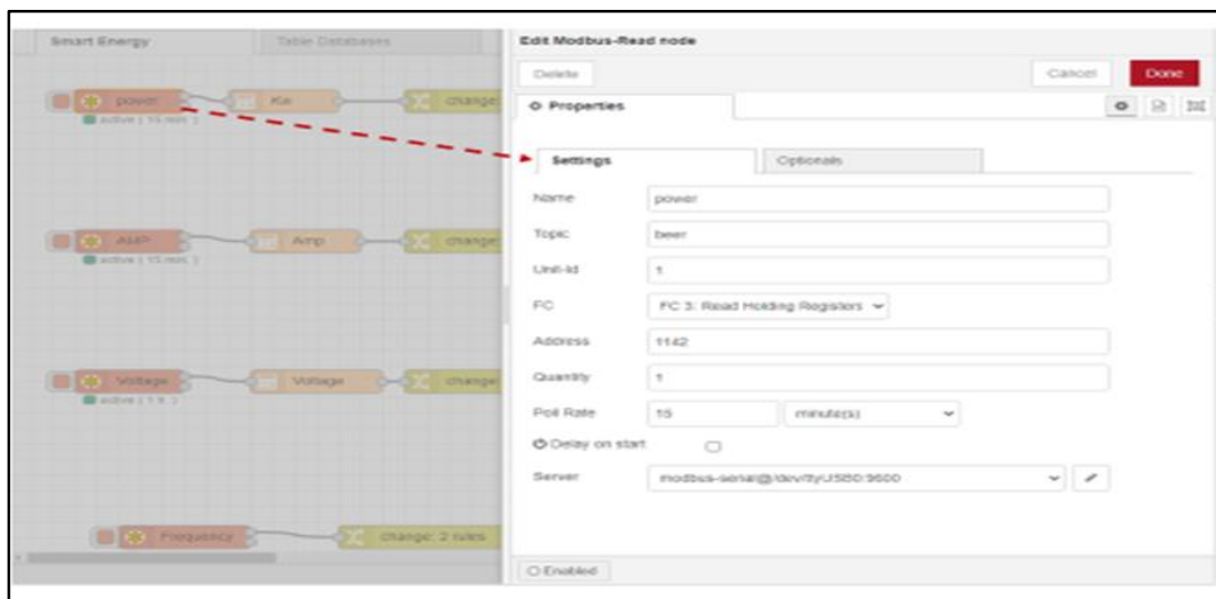
ภาพที่ 23 การตั้งค่าเชื่อมต่ออุปกรณ์ Multi-Function Digital Power Meter กับ SIEMENS SIMATIC IOT2050 ผ่านทางพอร์ต Serial RS-485 Protocol Modbus RTU
