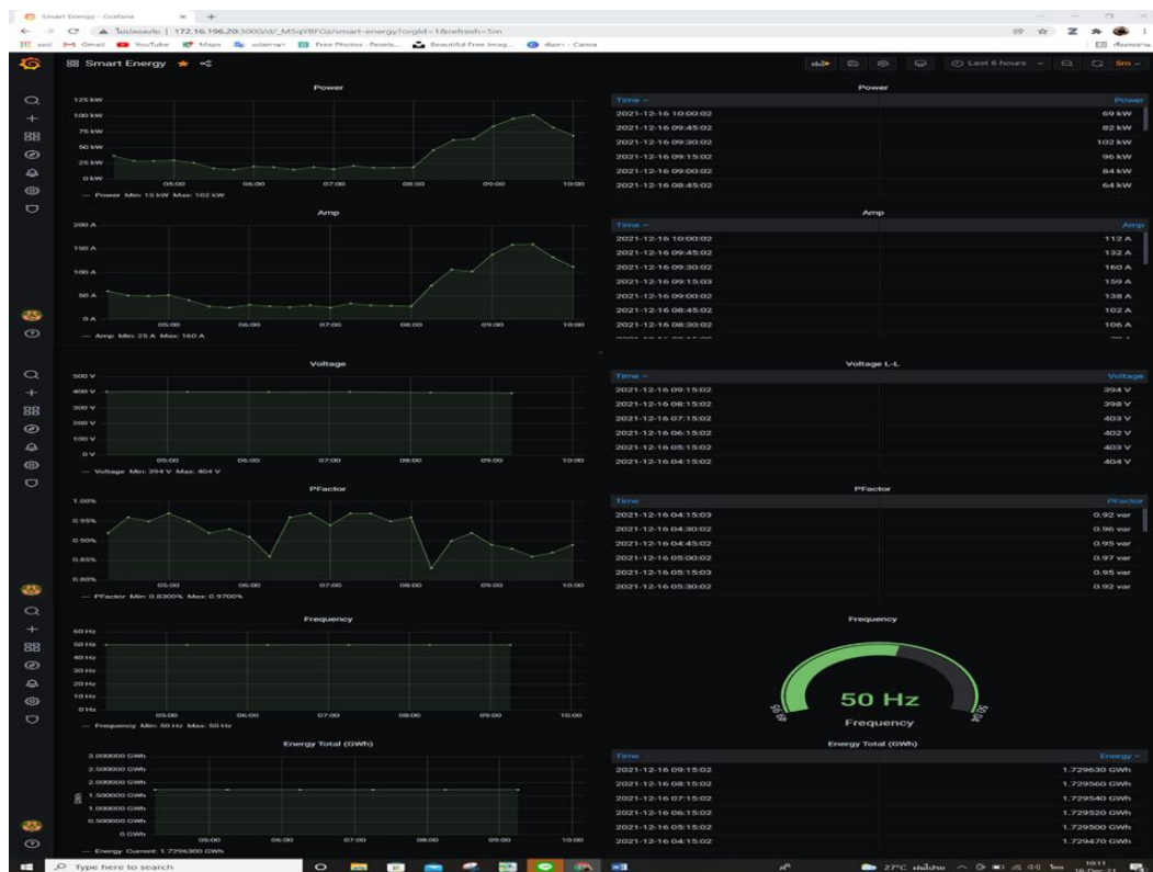
ภาพที่ 38 รูปแบบกราฟผ่านทาง Dashboard โปรแกรม Grafana
