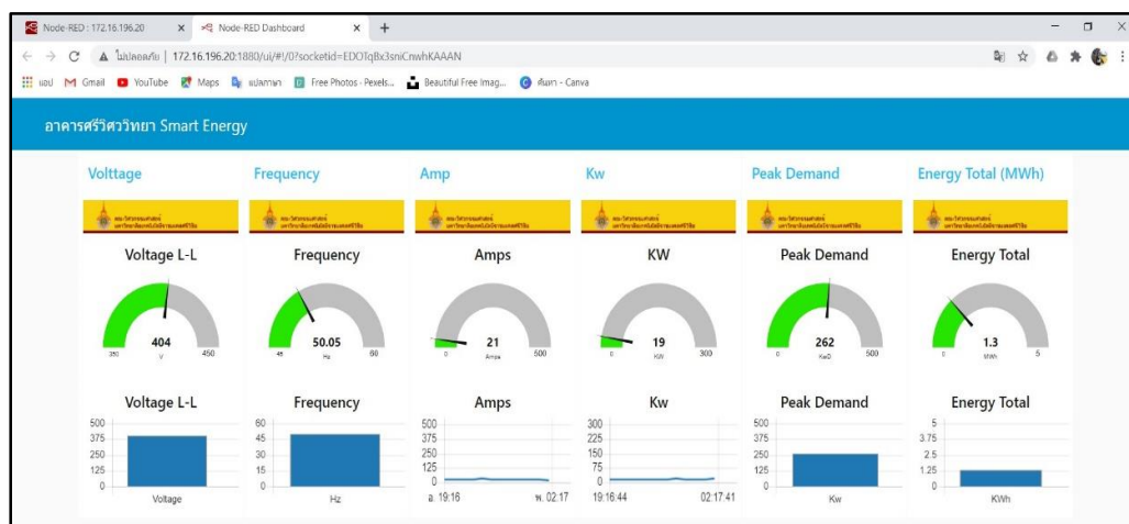
ภาพที่ 28 การสร้าง Node Dashboard สร้างและตั้งค่า Layout
