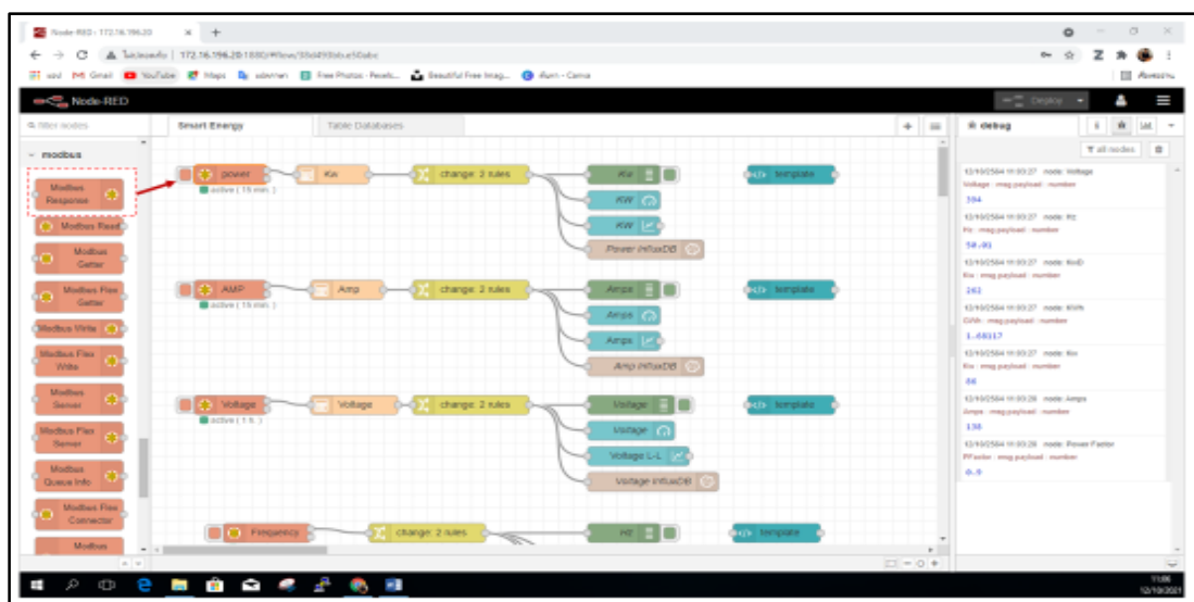
ภาพที่ 21 การสร้าง Node Modbus Read
