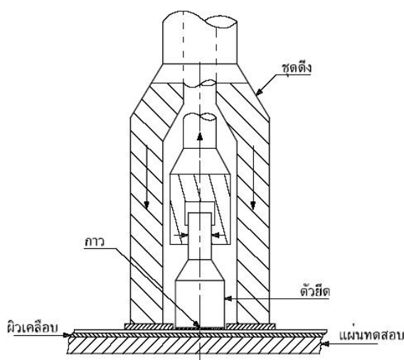
รูปที่ 2.8 การทดสอบการยึดติดของฟิล์ม โดยวิธีการดึง (Pull-off test)
