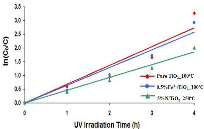
รูปที่ 3.33 กราฟความสัมพันธ์ระหว่าง \ln(C_0/C) กับเวลาในการรับแสง ภายใต้แสงยูวี ของฟิล์มไทเทเนียมไดออกไซด์สูตรต่างๆ ที่ดีที่สุดที่ความเข้มข้นเริ่มต้นของเมทิลีนบลู 10^{-6} โมลาร์
