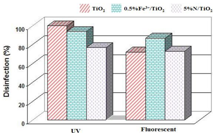
รูปที่ 3.37 เปอร์เซ็นต์การฆ่าเชื้อ E.coli ของฟิล์มไทเทเนียมไดออกไซด์สูตรต่างๆ ภายใต้แสงยูวี และแสงฟลูออเรสเซนต์ ที่เวลา 3 ชั่วโมง
