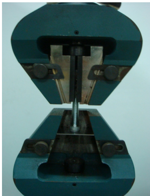
รูปที่ 3.39 การทดสอบความแข็งแรงของฟิล์มด้วยวิธีการดึง
