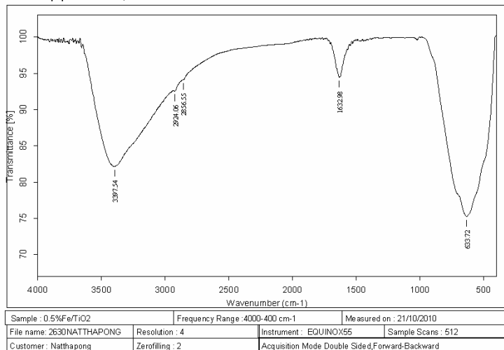
รูปที่ 3.22 FT-IR สเปกตรัมของผงไทเทเนียมไดออกไซด์ได้ปเหล็ก
