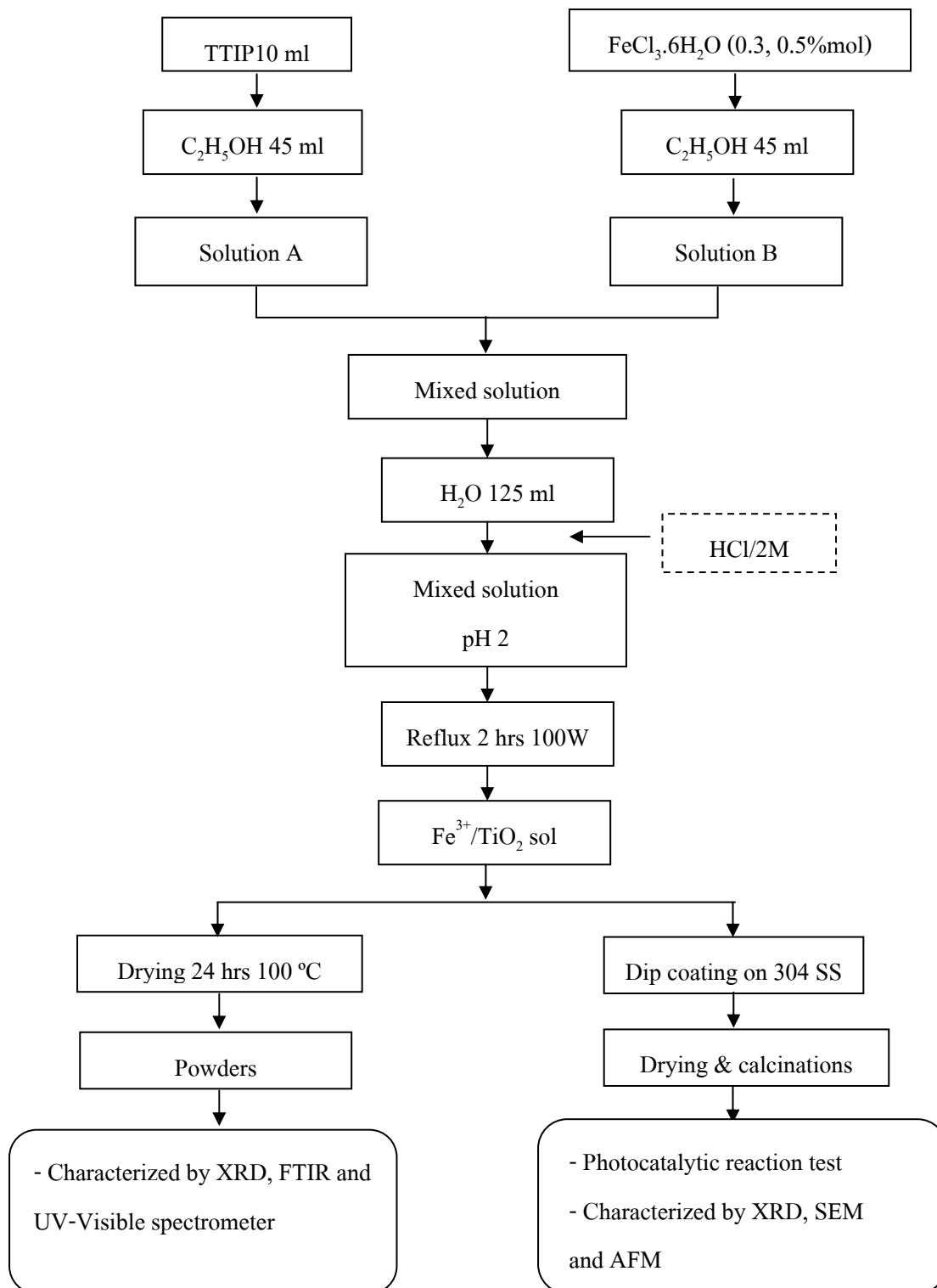
รูปที่ 2.2 การเตรียมผงและฟิล์มบางของไทเทเนียมไดออกไซด์ได้ปเหล็กด้วยวิธี โซล-เจล
