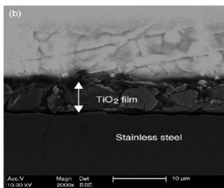
รูปที่ 1.11 फिल्मไทเทเนียมไดออกไซด์ที่เคลือบอยู่บนผิวของแผ่นเหล็กกล้าไร้สนิม
