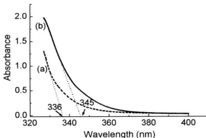
รูปที่ 2.7 การลากเส้นเพื่อหาค่าช่องว่างแถบพลังงาน (Band gap energy)
