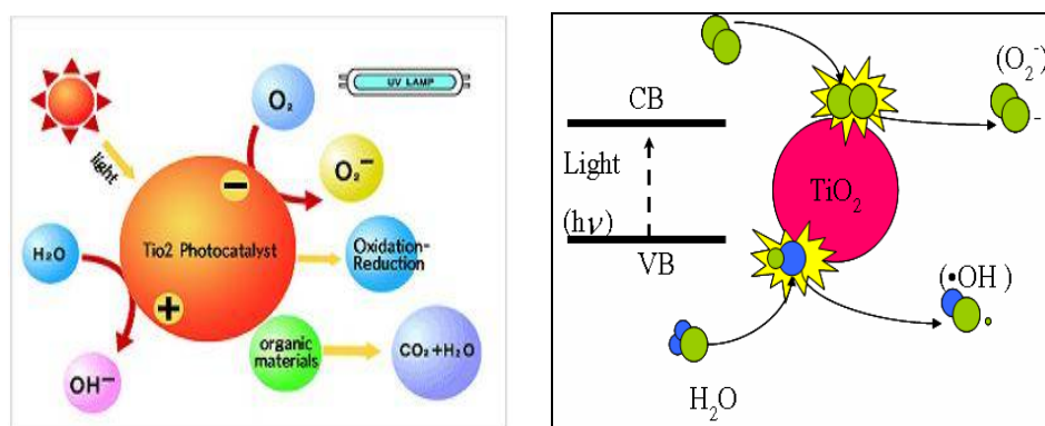
รูปที่ 1.4 กลไกการเกิดปฏิกิริยาโฟโตแคตะไลติก (Photocatalytic) ของไทเทเนียมไดออกไซด์
