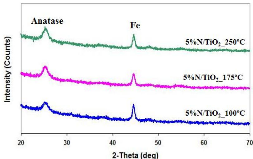
รูปที่ 3.10 ผล XRD ของฟิล์มไทเทเนียมไดออกไซด์ที่อบในโตรเจนที่เผาที่อุณหภูมิ 100 – 250 องศาเซลเซียส
