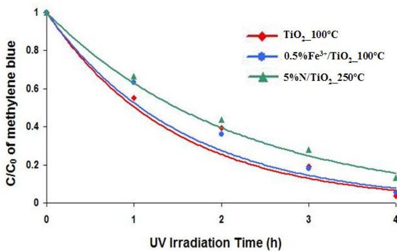
รูปที่ 3.30 ผลของปฏิกิริยาโฟโตแคตะไลติกของฟิล์มไทเทเนียมไดออกไซด์สูตรต่างๆ ที่ดีที่สุด ภายใต้แสงยูวีที่ความเข้มข้นเริ่มต้นของเมทิลีนบลู 10^{-6} โมลาร์
