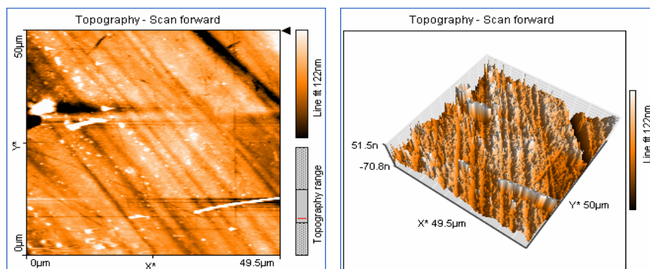
รูปที่ 3.19 ภาพถ่าย AFM ของไทเทเนียมไดออกไซด์ได้ป้เหล็ก
