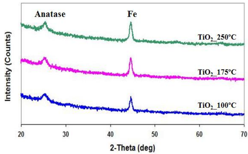
รูปที่ 3.8 ผล XRD ของฟิล์มไทเทเนียมไดออกไซด์ที่เผาที่อุณหภูมิ 100 – 250 องศาเซลเซียส
