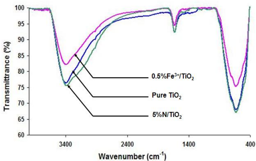
รูปที่ 3.24 FT-IR สเปกตรัมของผงไทเทเนียมไดออกไซด์สูตรต่างๆ
