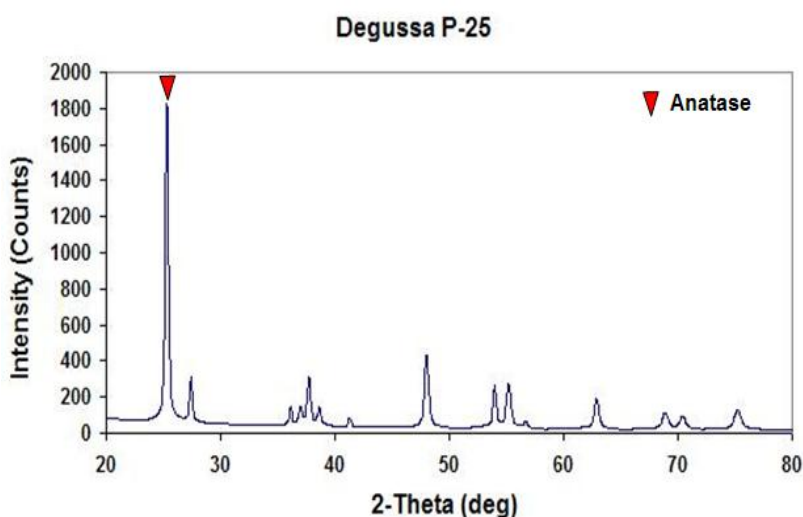
รูปที่ 3.5 ผล XRD ของผง Degussa P-25
