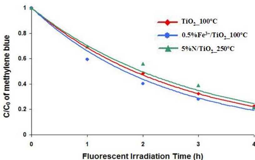
รูปที่ 3.31 ผลของปฏิกิริยาโฟโตแคตะไลติกของฟิล์มไทเทเนียมไดออกไซด์สูตรต่างๆ ที่ดีที่สุด ภายใต้แสงฟลูออเรสเซนซ์ที่ความเข้มข้นเริ่มต้นของเมทิลีนบลู 10^{-6} โมลาร์
