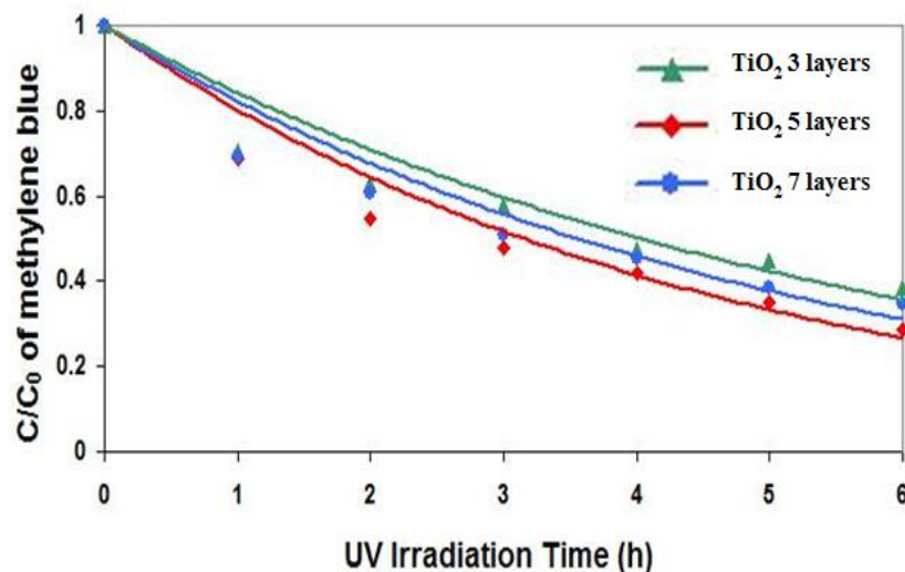
รูปที่ 3.14 ผลการทดสอบปฏิกิริยาโฟโตแคตะไลติกของฟิล์มไทเทเนียมไดออกไซด์ที่จำนวนชั้นเคลือบ 3, 5 และ 7 ชั้น
