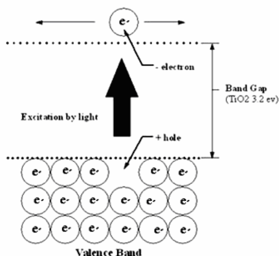
รูปที่ 1.3 กระบวนการที่เกิดขึ้นเมื่อสารกึ่งตัวนำไทเทเนียมไดออกไซด์ถูกกระตุ้นด้วยแสง (ที่มา: http://www.vcharkarn.com/varticle/27809 : 12/02/2554)
