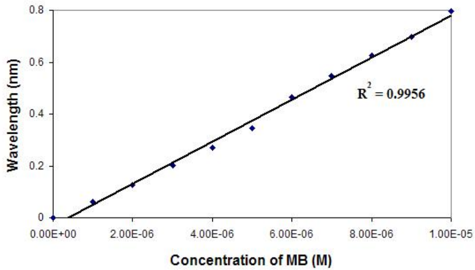
รูปที่ 2.5 ความสัมพันธ์ระหว่างความเข้มข้นของสารละลายเมทิลีนบลู 1 \times 10^{-6} - 1 \times 10^{-5} โมลาร์ กับค่า Absorbance ที่ได้จากเครื่อง UV-VIS spectrophotometer
