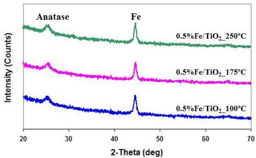
รูปที่ 3.9 ผล XRD ของฟิล์มไทเทเนียมไดออกไซด์ที่เติมด้วยเหล็กที่เผาที่อุณหภูมิ 100 – 250 องศาเซลเซียส
