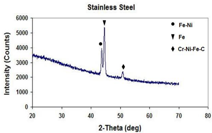
รูปที่ 3.7 ผล XRD ของชิ้นงานทดสอบ (304 Stainless Steel)
