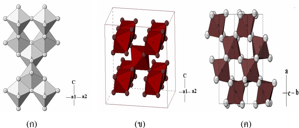
รูปที่ 1.2 โครงสร้างผลึกของเฟสไทเทเนียมไดออกไซด์ (ก) อะนาเทส (ข) รูไทล์ (ค) บรูคไคต์ (ที่มา: http://staff.aist.go.jp/nomura-k/english/itscgallery-e.htm : 12/02/2554)
