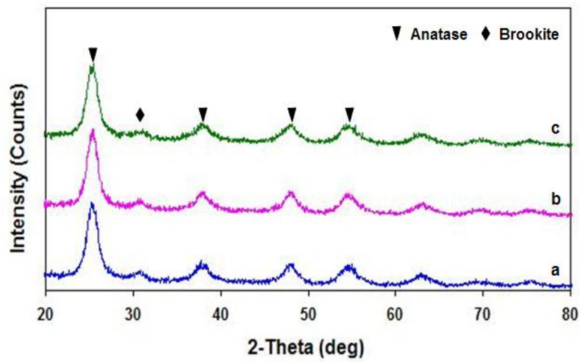
รูปที่ 3.6 ผล XRD ของผงไทเทเนียมไดออกไซด์ a) \text{TiO}_2 , b) 0.5\%\text{Fe}^{3+}/\text{TiO}_2 และ c) 5\%\text{N}/\text{TiO}_2
