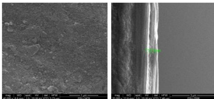
รูปที่ 3.15 ภาพถ่าย SEM ของพื้นผิวของฟิล์มและความหนาของฟิล์มของไทเทเนียมไดออกไซด์
