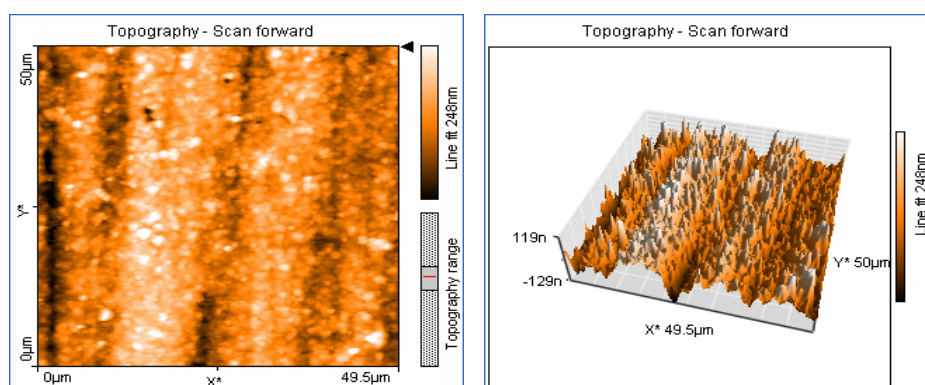
รูปที่ 3.20 ภาพถ่าย AFM ของไทเทเนียมไดออกไซด์ได้ป้ใน โตรเจน
