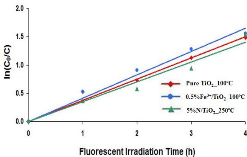
รูปที่ 3.34 กราฟความสัมพันธ์ระหว่าง \ln(C_0/C) กับเวลาในการรับแสง ภายใต้แสงฟลูออเรสเซนซ์ของฟิล์มไทเทเนียมไดออกไซด์สูตรต่างๆ ที่ดีที่สุดที่ความเข้มข้นเริ่มต้นของเมทิลีนบลู 10^{-6} โมลาร์
