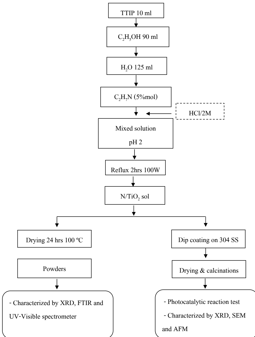
รูปที่ 2.3 การเตรียมผงและฟิล์มบางของไทเทเนียมไดออกไซด์โด๊ปไนโตรเจนด้วยวิธี โซล-เจล
