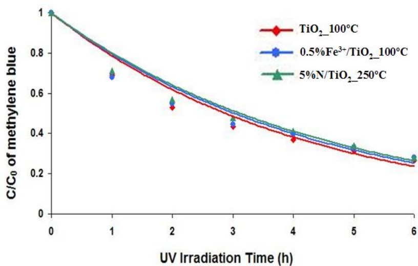
รูปที่ 3.29 ผลของปฏิกิริยาโฟโตแคตะไลติกของฟิล์มไทเทเนียมไดออกไซด์สูตรต่างๆ ที่ดีที่สุด ภายใต้แสงยูวีที่ความเข้มข้นเริ่มต้นของเมทิลีนบลู 10^{-5} โมลาร์
