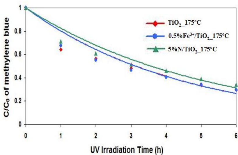
รูปที่ 3.27 ผลการทดสอบปฏิกิริยาโฟโตแคตะไลติกของฟิล์มไทเทเนียมไดออกไซด์สูตรต่างๆ ภายใต้แสงยูวีที่อุณหภูมิในการเผา 175 องศาเซลเซียส ที่ความเข้มข้นเริ่มต้น 10^{-5} โมลาร์
