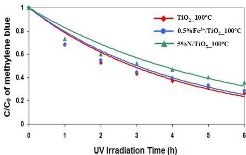
รูปที่ 3.26 ผลการทดสอบปฏิกิริยาโฟโตแคตะไลติกของฟิล์มไทเทเนียมไดออกไซด์สูตรต่างๆ ภายใต้แสงยูวีที่อุณหภูมิในการเผา 100 องศาเซลเซียส ที่ความเข้มข้นเริ่มต้น 10^{-5} โมลาร์
