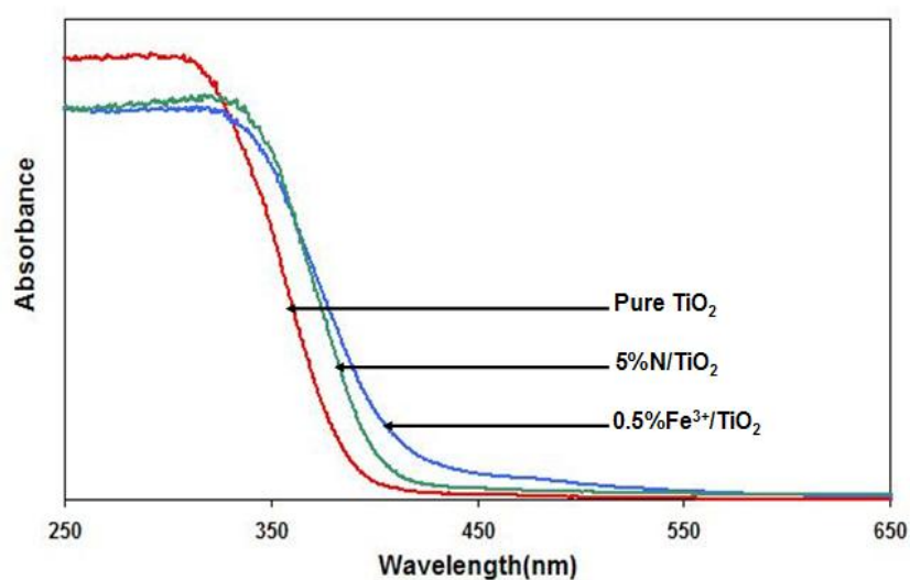
รูปที่ 3.25 ผล UV-VIS ของผงไทเทเนียมไดออกไซด์สูตรต่างๆ
