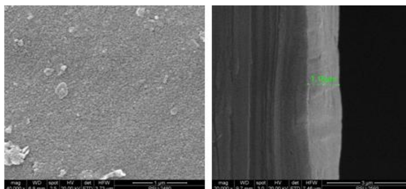
รูปที่ 3.17 ภาพถ่าย SEM ของพื้นผิวของฟิล์มและความหนาของฟิล์มของไทเทเนียมไดออกไซด์ ได้ปไนโตรเจน
