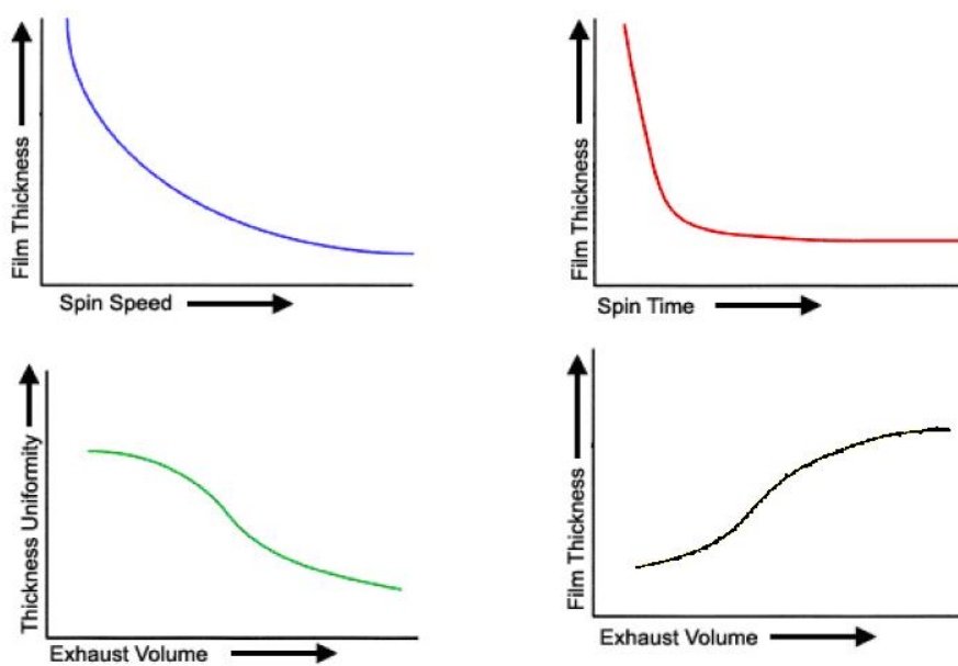
รูปที่ 1.9 ความสัมพันธ์ระหว่างความหนาของฟิล์มกับความเร็ว เวลาและปริมาณของสารละลายที่ใช้ในการหมุนเหวี่ยง
