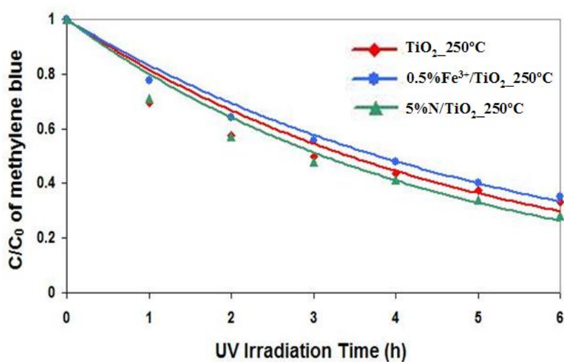
รูปที่ 3.28 ผลการทดสอบปฏิกิริยาโฟโตแคตะไลติกของฟิล์มไทเทเนียมไดออกไซด์สูตรต่างๆ ภายใต้แสงยูวีที่อุณหภูมิในการเผา 250 องศาเซลเซียส ที่ความเข้มข้นเริ่มต้น 10^{-5} โมลาร์
