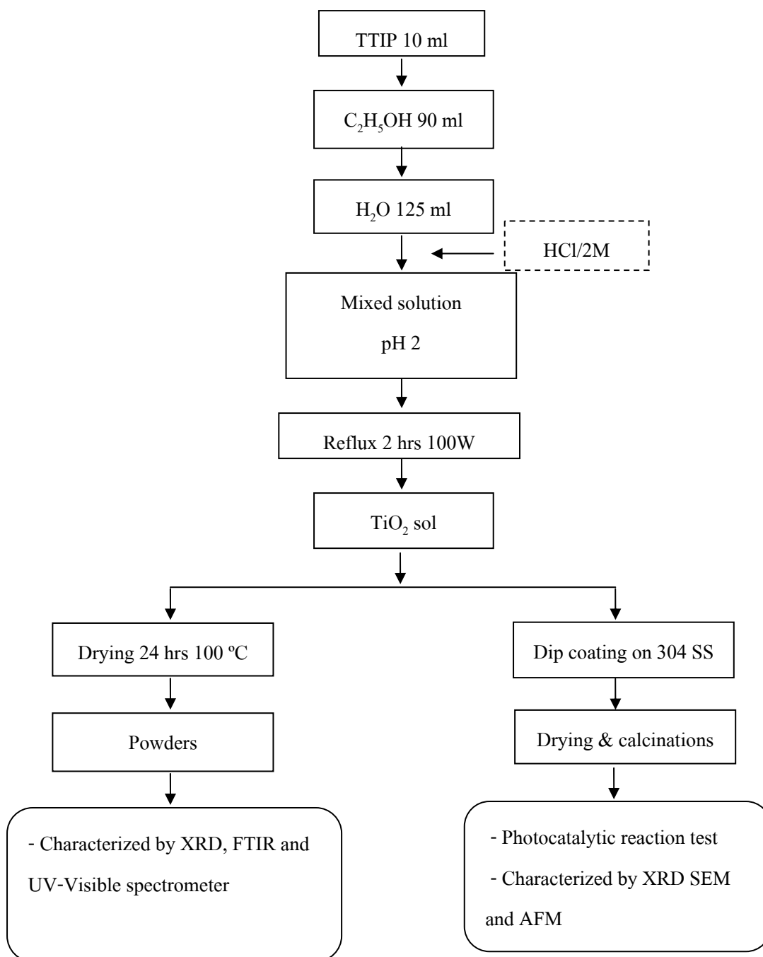
รูปที่ 2.1 การเตรียมผงและฟิล์มบางของไทเทเนียมไดออกไซด์ด้วยวิธี โซล-เจล
