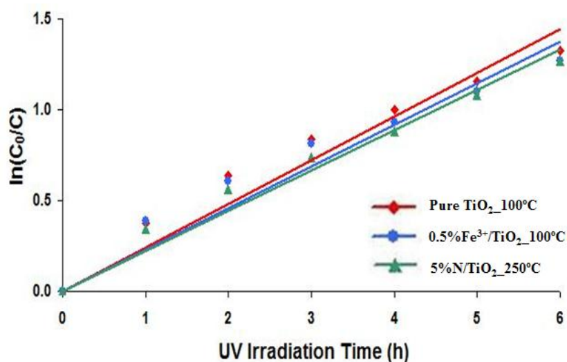
รูปที่ 3.32 กราฟความสัมพันธ์ระหว่าง \ln(C_0/C) กับเวลาในการรับแสง ภายใต้แสงยูวี ของฟิล์ม ไทเทเนียมไดออกไซด์สูตรต่างๆ ที่ดีที่สุดที่ความเข้มข้นเริ่มต้นของเมทิลีนบลู 10^{-6} โมลาร์
