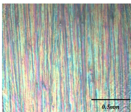
รูปที่ 3.11 ภาพถ่ายพื้นผิวของฟิล์มไทเทเนียมไดออกไซด์ที่จำนวนชั้นเคลือบ 3 ชั้น
