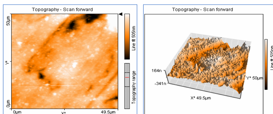
รูปที่ 3.18 ภาพถ่าย AFM ของไทเทเนียมไดออกไซด์
