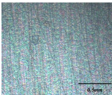
รูปที่ 3.12 ภาพถ่ายพื้นผิวของฟิล์มไทเทเนียมไดออกไซด์ที่จำนวนชั้นเคลือบ 5 ชั้น
