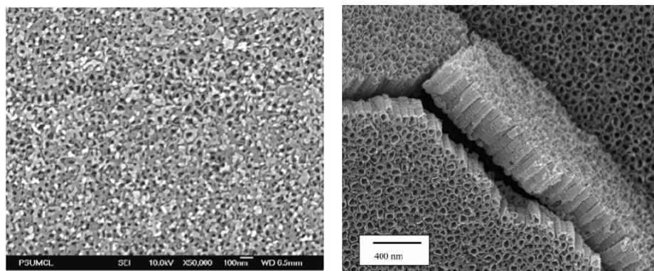
รูปที่ 1.13 ภาพถ่าย FESEM ของ \text{TiO}_2 Nanotube arrays (ที่มา: Gopal, et al., 2006)
