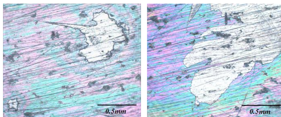
รูปที่ 3.40 ลักษณะการหลุดลอกของผิวฟิล์มหลังการทดสอบความแข็งแรงของฟิล์มด้วยวิธีการดึง
