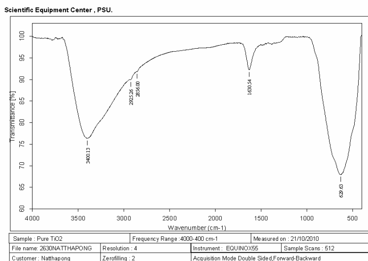
รูปที่ 3.21 FT-IR สเปกตรัมของผงไทเทเนียมไดออกไซด์
